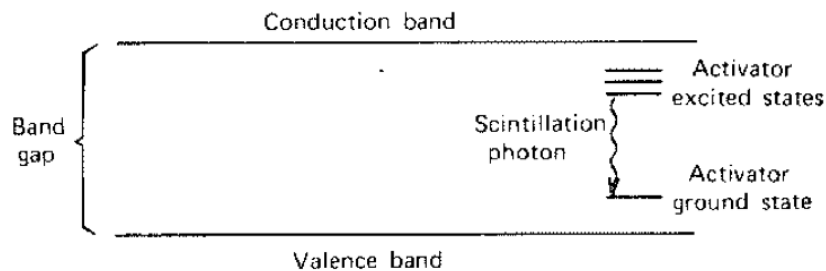
Figura 3.3 - Estrutura de bandas de energia de um cintilador cristilino ativado. Fonte: Knoll (1989).
