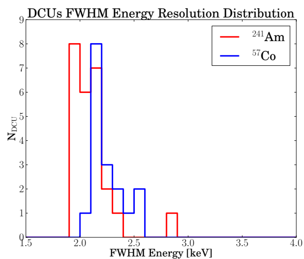
Figura 5.15 - Distribuição de valores médios da resolução em energia FWHM de 17 DCUs testadas com 57 Co (azul) e de 25 DCUs testadas com 241 Am (vermelho). A mediana (FWHM) obtida para a linha de 122 keV é 2.27 \pm 0.74 keV, enquanto para a linha de 59.6 keV é 2.12 \pm 0.18 keV. Fonte: Rodrigues et al. (2013).
