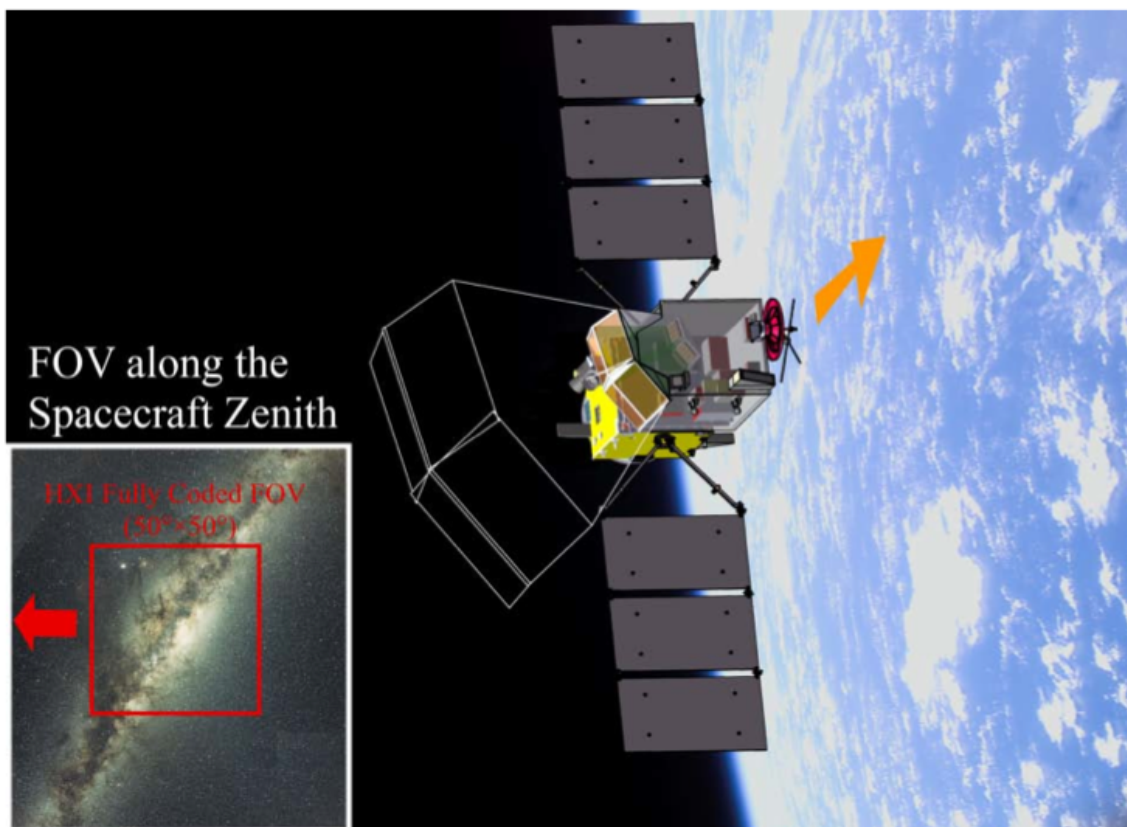
Figura 4.3 - Visão artística do satélite Lattès, que é baseado na Plataforma Multi-Missão (PMM). Os 4 telescópios de raios X duros do MIRAX são mostrados no módulo de carga-útil. Fonte: Grindlay e Bonnenfant (2011).
