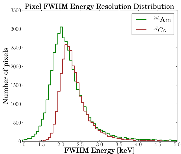
Figura 5.14 - Distribuição de resolução em energia FWHM de todos os pixels de 25 DCUs testados com 241 Am (verde) e 17 DCUs testadas com 57 Co (marrom).
