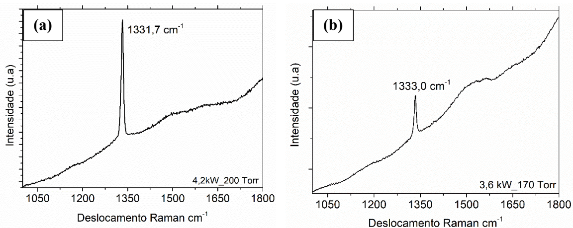
Figura 2. Espectroscopia de espalhamento Raman para MCD. (a) porta-substrato A. (b) porta-substrato B. Fonte: produção do autor.
