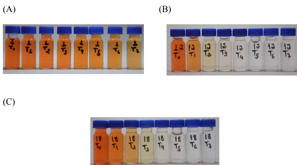
Figura 5.3 - Imagens das soluções do RO16 eletrolisadas a 25 \text{ mA cm}^{-2} com os eletrodos (A) 5.000 ppm (B) 15.000 ppm e (C) 30.000 ppm, em função do tempo de eletrólise.
