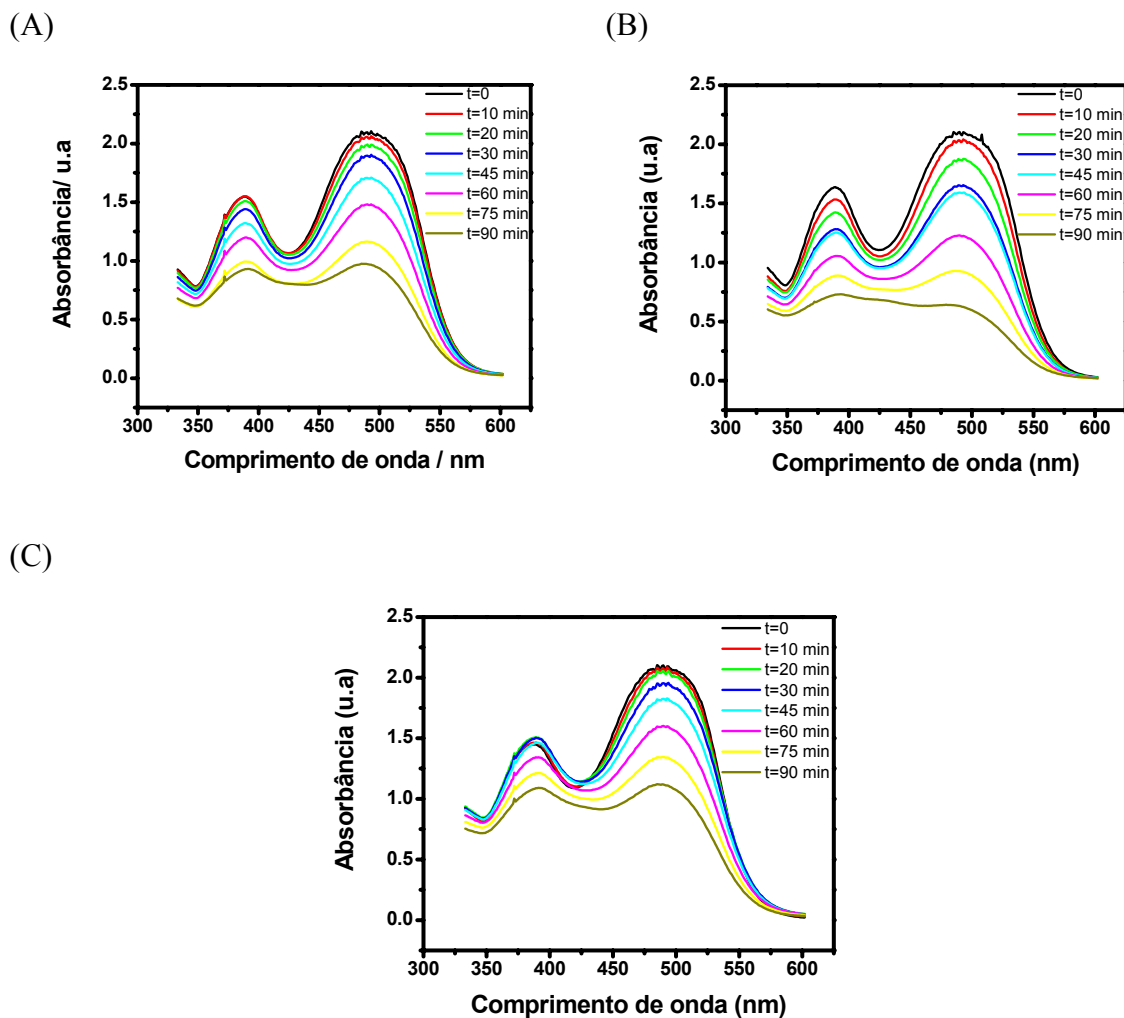
Figura 5.1 - Espectros de absorção das soluções de RO16 eletrolisas a 25 \text{ mA cm}^{-2} com os eletrodos (A) 5.000 ppm (B) 15.000 ppm e (C) 30.000 ppm, entre 300 e 600 nm, em função do tempo de eletrólise.
