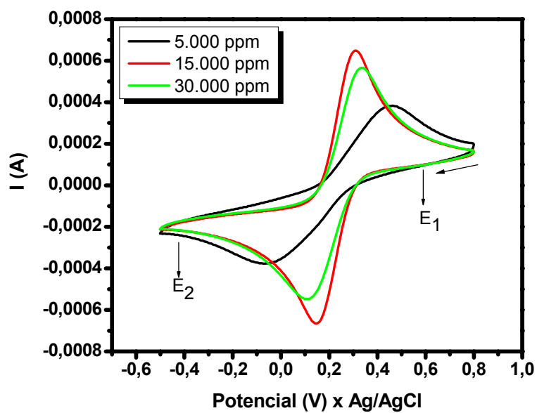
Figura 4.11 - Voltamogramas cíclicos em 0,1 \text{ mol L}^{-1} \text{ KCl} + 1 \text{ mmol L}^{-1} \text{ K}_3\text{Fe}(\text{CN})_6 e v = 30 \text{ mV s}^{-1} para os eletrodos de diamante dopado em diferentes níveis de boro, com um tempo de deposição de 7h.
