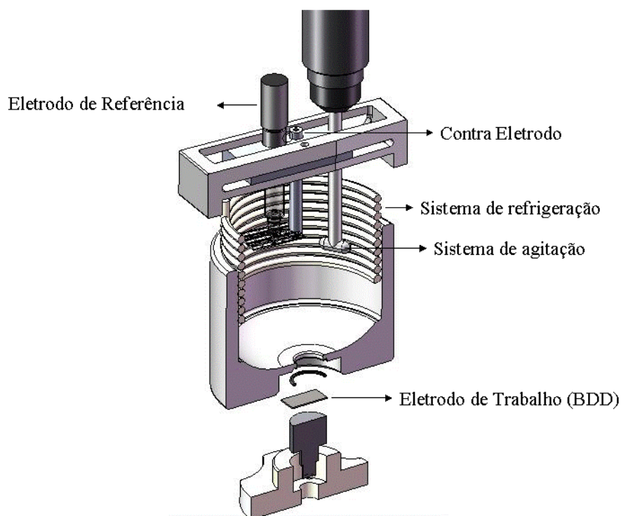
Figura 3.2 - Célula eletroquímica
