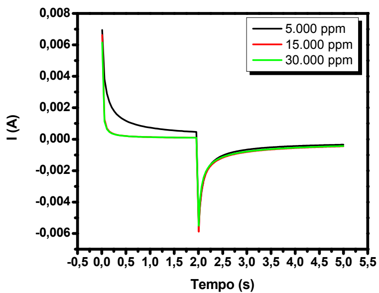
Figura 4.13 - Ensaio cronamperométrico do tipo “ potential-step ”, em função do tempo de deposição dos filmes de 7h.
