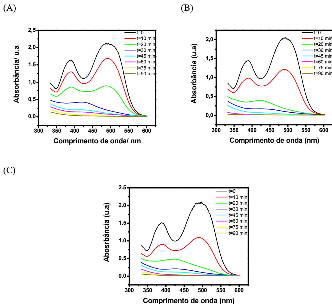
Figura 5.2 - Espectros de absorção das soluções de RO16 eletrolisadas a 200 \text{ mA cm}^{-2} com os eletrodos (A) 5.000 ppm (B) 15.000 ppm e (C) 30.000 ppm, entre 300 e 600 nm, em função do tempo de eletrólise.
