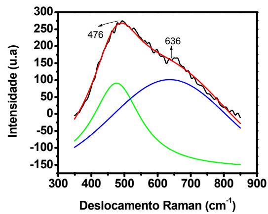
Figura 4.5 - Exemplos de ajuste do pico de 500 cm -1 por uma componente Lorentziana e uma Gaussiana, para as amostras de 5.000, 15.000 e 30.000 ppm para os crescimentos de 7 h.
