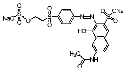
Figura 2.1- Fórmula Estrutural do corante reativo alaranjado 16 (RO16).
