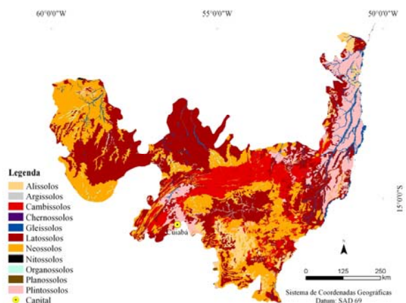
Fig. 8 – Mapa de solos da área de estudo.
