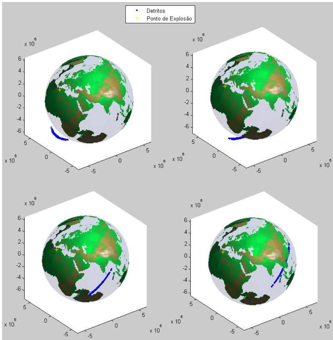
Figura A.59 – Distribuição de Detritos no 5º Caso com Parâmetros CR = 0,5 , CS = 0,5 e \sigma_v = 50 m/s nos instantes 1,2P_{sat} , 1,3P_{sat} , 1,4P_{sat} e 1,5P_{sat} .
