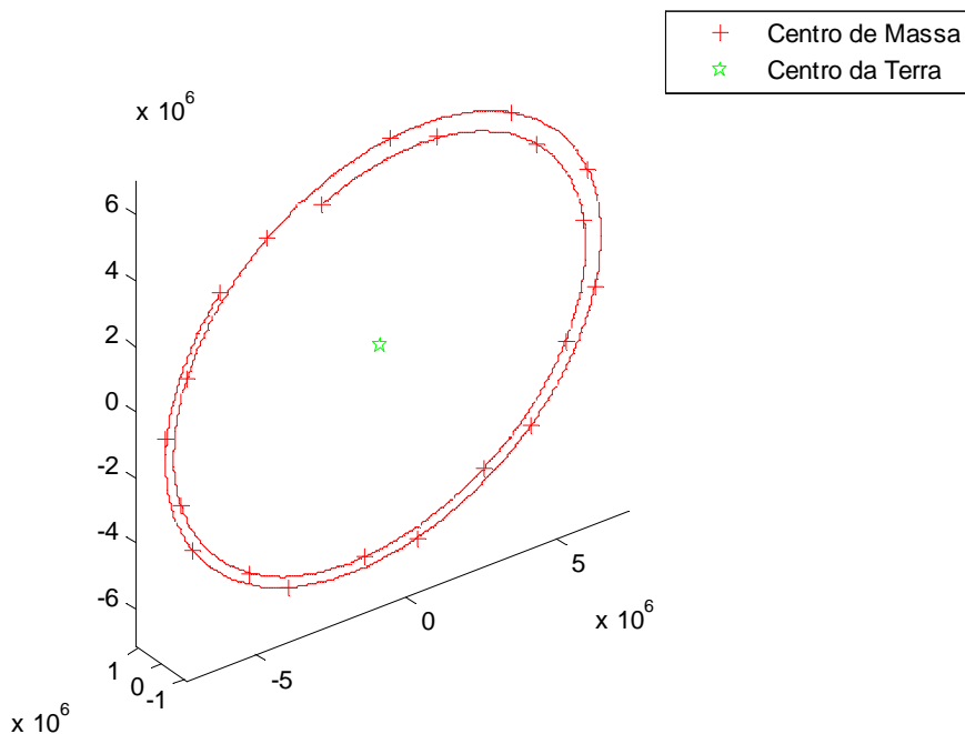
Figura 4.44 – Centro de Massa da Distribuição de Detritos no 6º Caso com Parâmetros CR = 0,5 e \sigma_v = 100 m/s.
