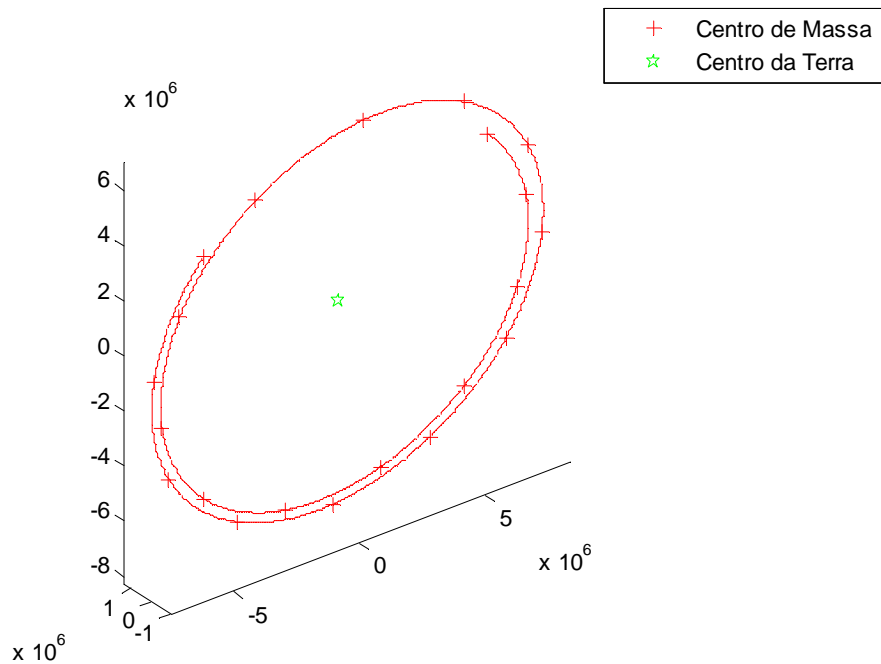
Figura 4.26 – Centro de Massa da Distribuição de Detritos no 5º Caso com Parâmetros CR = 1 e \sigma_v = 100 m/s.
