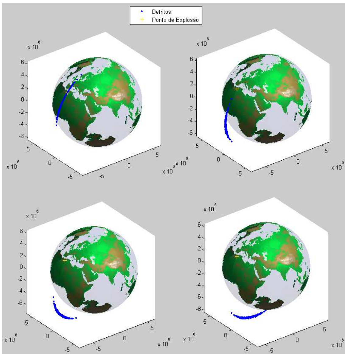
Figura A.79 – Distribuição de Detritos no 5º Caso com Parâmetros CR = 0,5 , CS = 0,5 e \sigma_v = 100 m/s nos instantes 1,2P_{sat} , 1,3P_{sat} , 1,4P_{sat} e 1,5P_{sat} .
