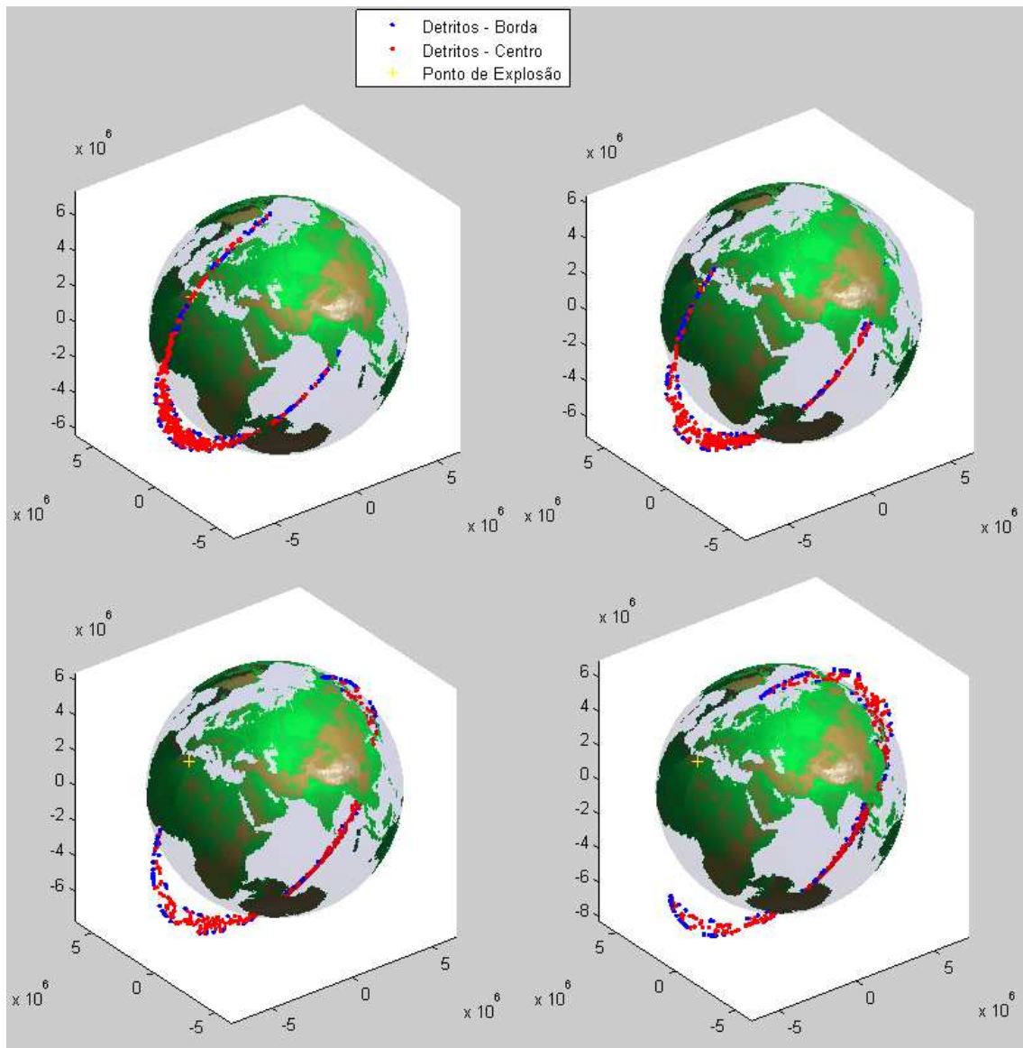
Figura A.9 – Distribuição de Detritos no 1º Caso com Parâmetros \beta = 200 e r = 3 m nos instantes 1,2P_{sat} , 1,3P_{sat} , 1,4P_{sat} e 1,5P_{sat} .
