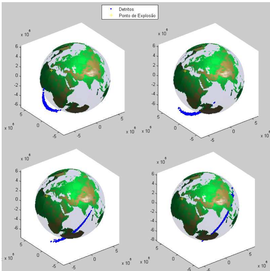
Figura A.114 – Distribuição de Detritos no 6º Caso com Parâmetros CR = 1 , CS = 1 e \sigma_v = 100 m/s nos instantes 1,2P_{\text{sat}} , 1,3P_{\text{sat}} , 1,4P_{\text{sat}} e 1,5P_{\text{sat}} .
