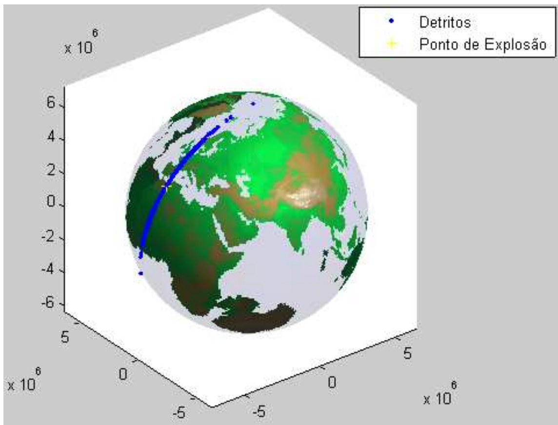
Figura 4.9 – Distribuição de Detritos no 3º Caso com Parâmetro \sigma_v = 50 m/s no instante 2P_{sat} .
