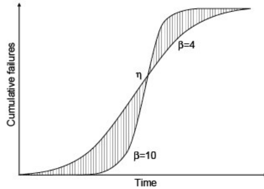
Figura 3- Falhas cumulativas como uma função do tempo pela distribuição de Weibull de 2 parâmetros. Fonte: SARKKA (2008)
