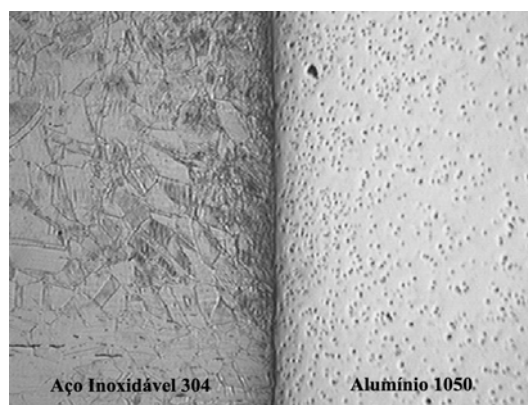
Figura 8 – Fotomicrografia da interface de soldagem entre a liga de alumínio AA 1050 e o aço inoxidável AISI 304 com aumento de 100 X.
