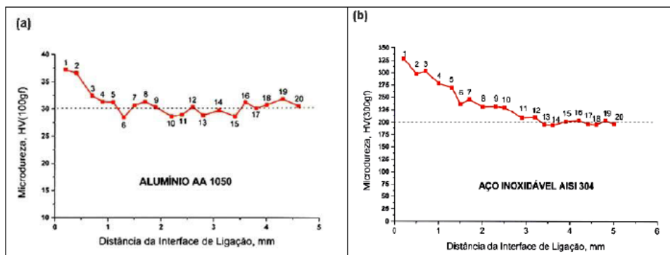
Figura 7 – Gráfico Microdureza HV x Distância da Interface de Ligação – (a) alumínio AA 1050; (b) aço inoxidável AISI 304.
