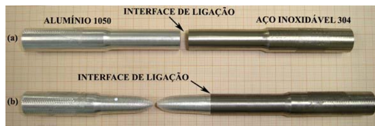
Figura 6 – Corpo de prova N° 5 (a) – ruptura na interface; corpo de prova N° 8 (b) – ruptura longe da interface de ligação.
