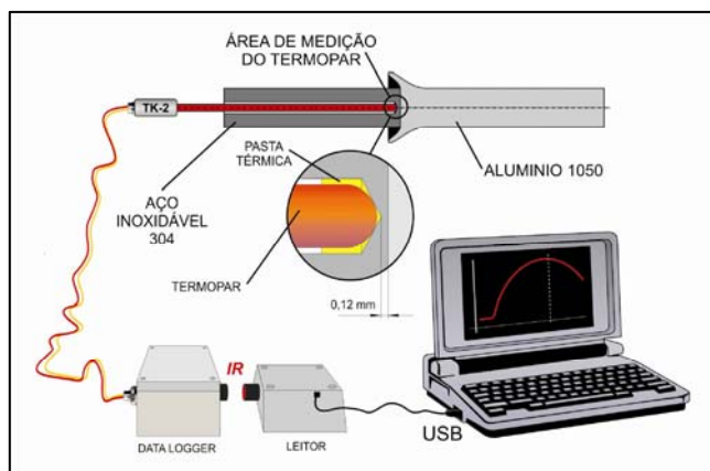
Figura 4 – Sistema TDL composto de termopar tipo K, Data Logger, leitor IR (infravermelho) e notebook para monitoramento da temperatura.
