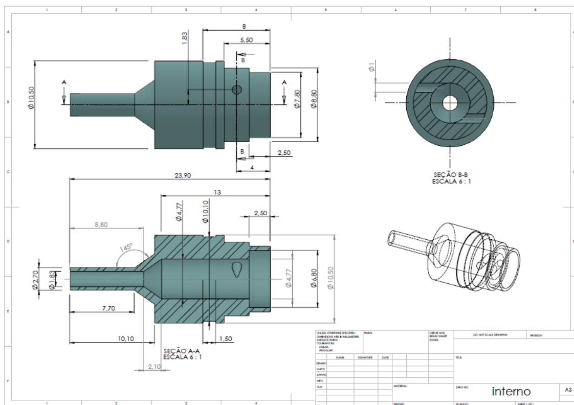
Figura D.1 - Esquema da câmara primária do injetor centrífugo dual.
