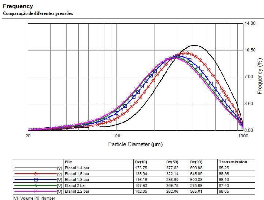
Figura 8.16 - Funções densidade de probabilidade (frequência) dos diâmetros das gotas formadas pela injeção de etanol hidratado na câmara primária para diferentes pressões de injeção (manométricas).
