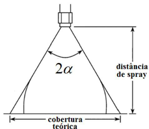
Figura 6.1 - Definição do ângulo de cone.
