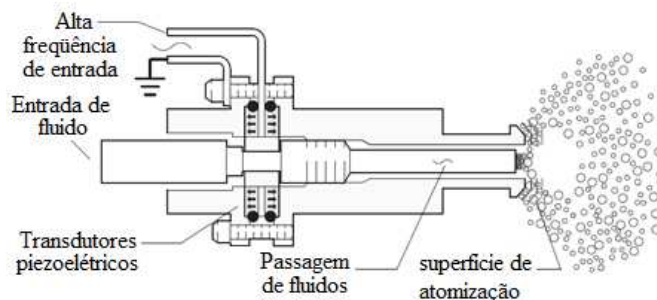
Figura 2.6 - Atomizador ultra-sônico.
