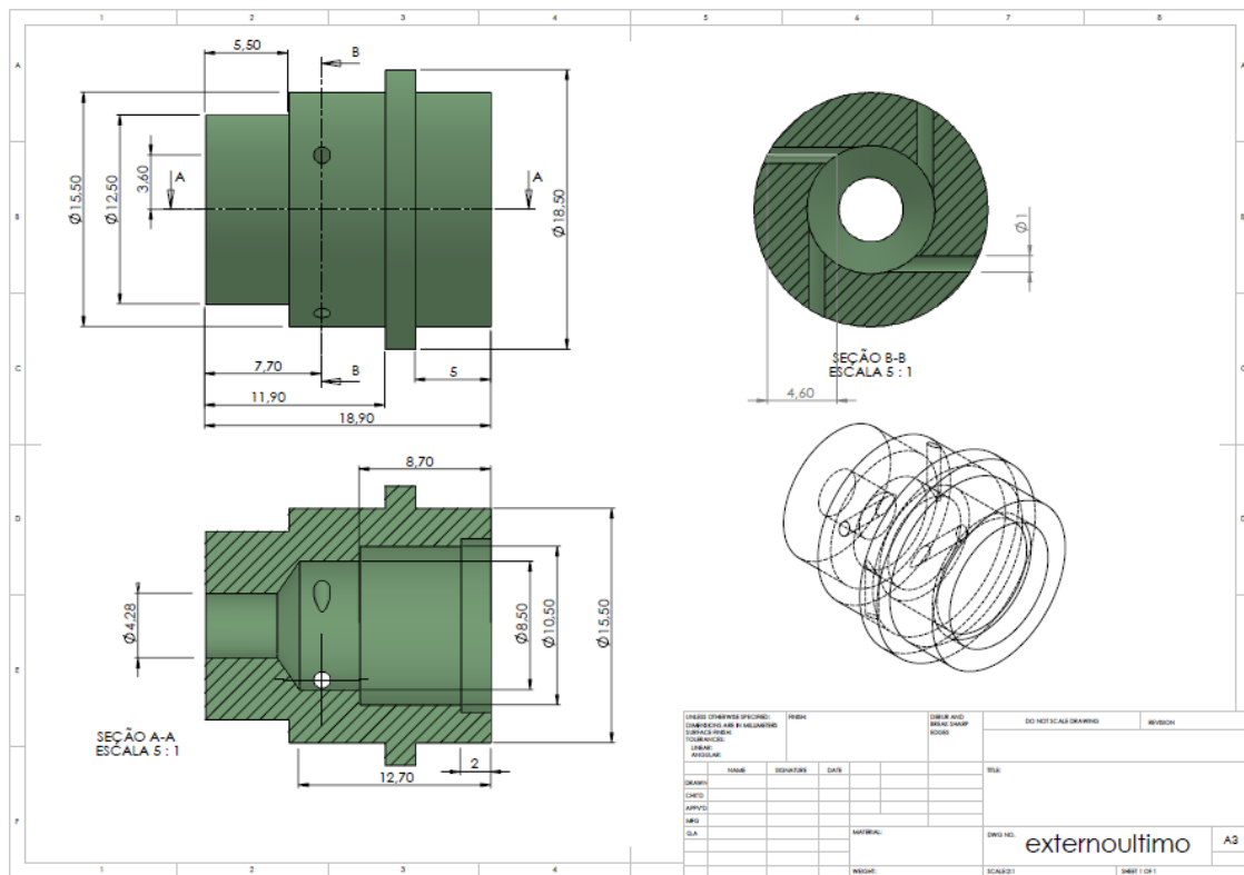
Figura D.2 - Esquema da câmara secundária do injetor centrífugo dual.
