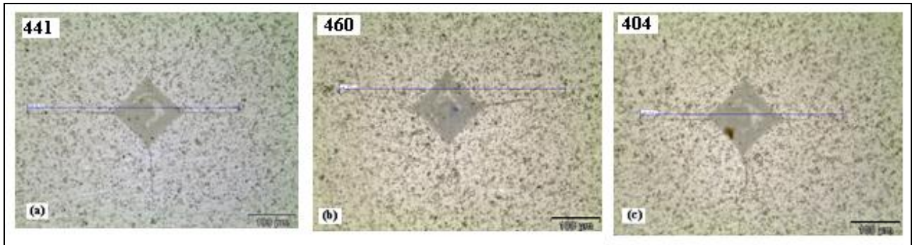
Figura 4.18 - Imagens obtidas por microscopia ótica mostrando as trincas geradas pela penetração Vickers em 3 regiões na cerâmica da composição C.
