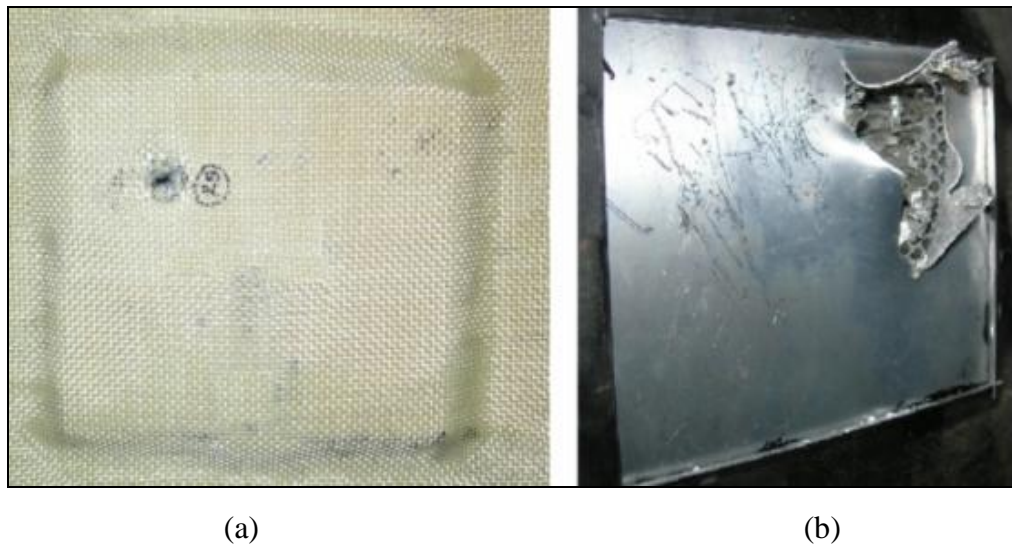
Figura 4.25 – Ensaio da blindagem 1, impactadas por projétil .44 Magnum: (a) vista do impacto frontal e (b) vista traseira da placa.
