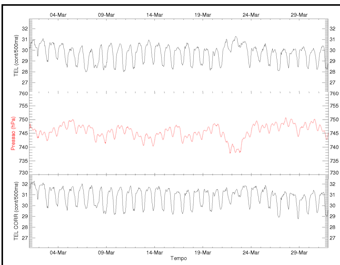
Figura 3.5 – No gráfico superior: contagem de raios cósmicos registrada pelo sinal TELESOCPE do detector CARPET no mês de Março de 2010. A curva vermelha representa a pressão atmosférica registrada no mesmo período e no gráfico inferior é mostrada a contagem corrigida pela pressão.
