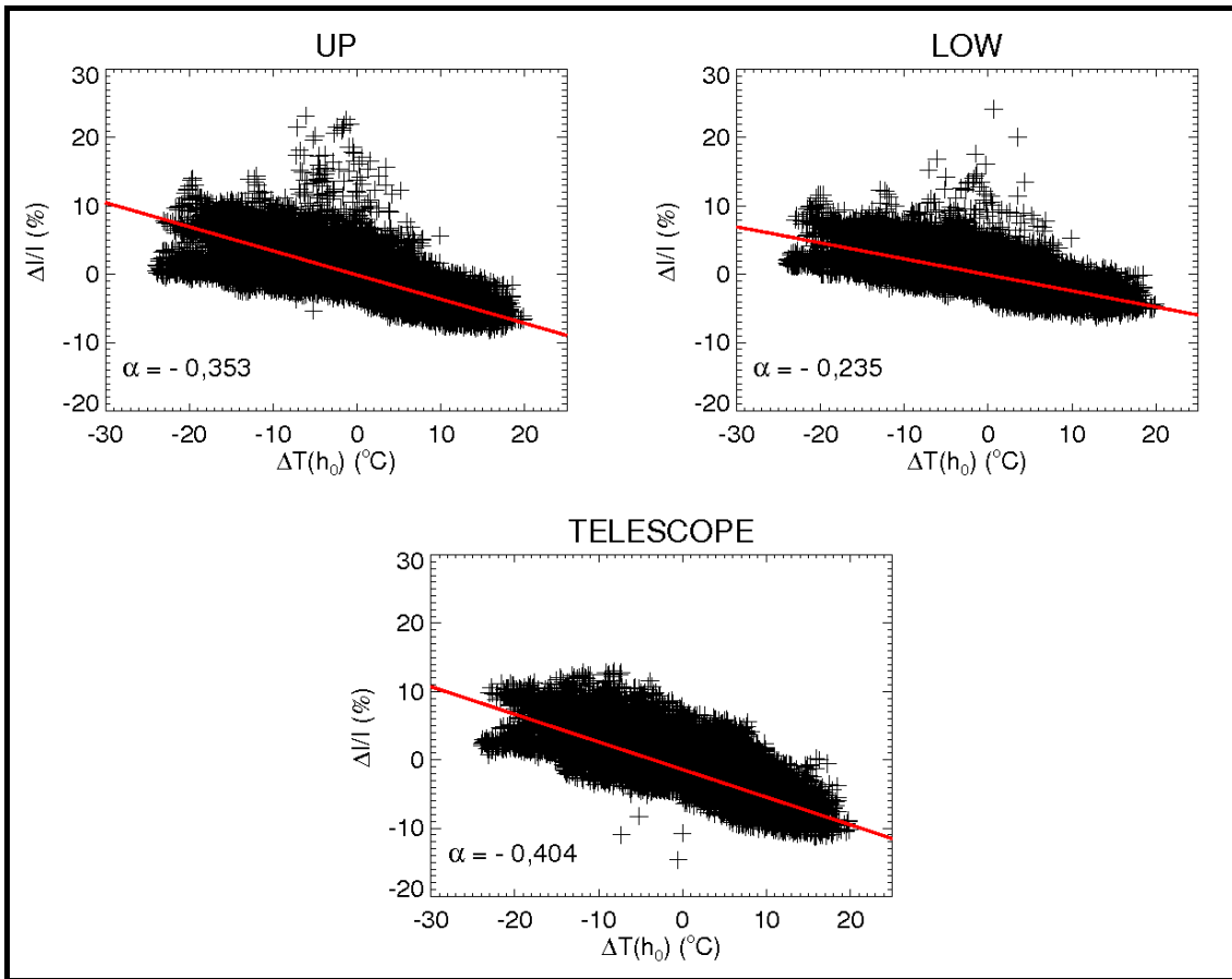
Figura 3.7 – Anticorrelações obtidas através da análise da variação relativa da contagem de raios cósmicos ( \Delta I/I ) observada, entre Abril de 2006 e Agosto de 2010, em cada um dos três sinais do CARPET e a variação de temperatura registrada na superfície ( \Delta T(h_0) ).
