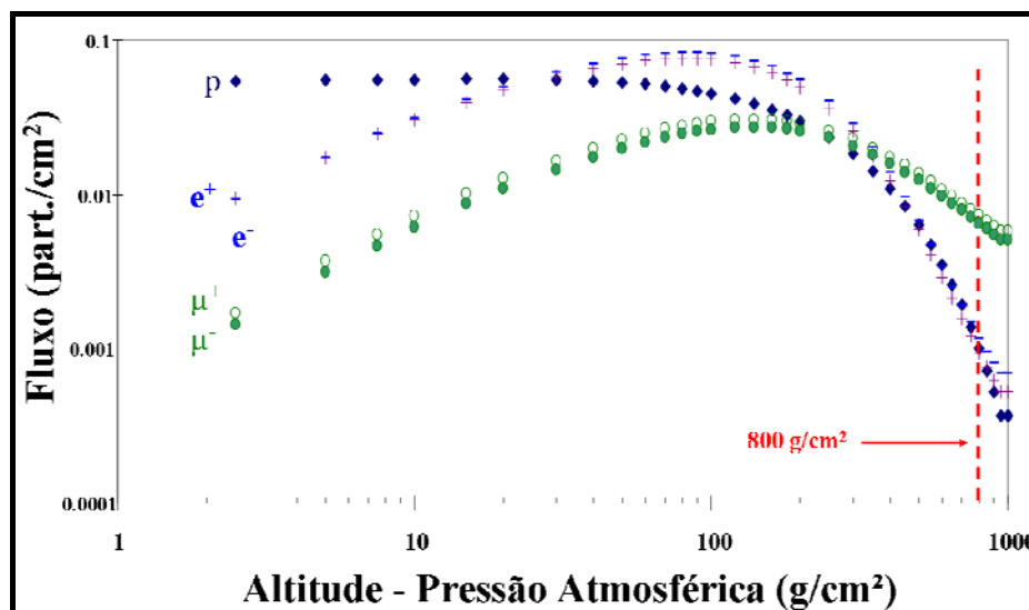
Figura 2.10 – Variação do fluxo dos múons negativos e positivos (pontos verdes), dos pósitrons (sinal de “+”), dos elétrons (sinal de “-”) e dos prótons (losango azul) com a altitude calculada através de experimentos com balões
