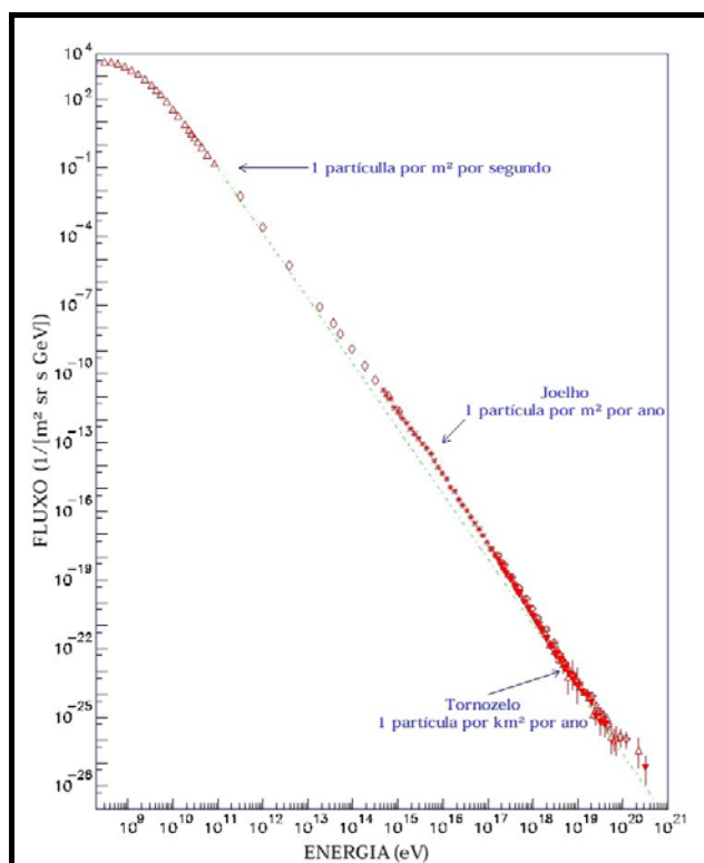
Figura 2.1 – Espectro de Energia dos Raios C3smicos Gal3cticos.
