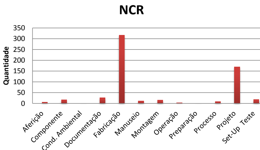
Figura 5.2 - Origem das NCR's (CBERS-1&2).
