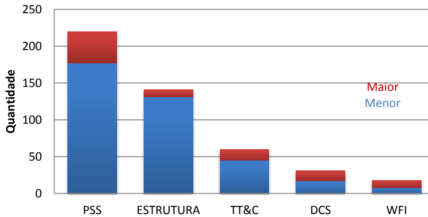
Figura 5.4 - NCR's do satélite CBERS-1.
