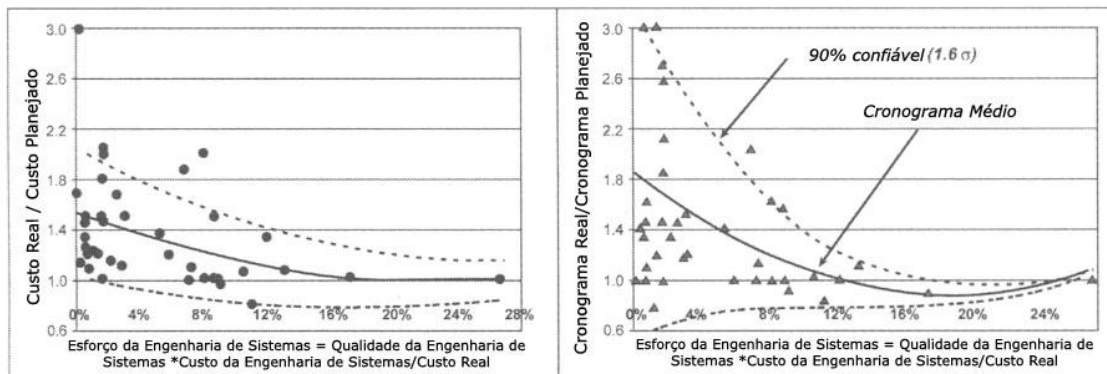
Figura 2.3 - Custo e cronograma correlacionados com o esforço da engenharia de sistemas.
