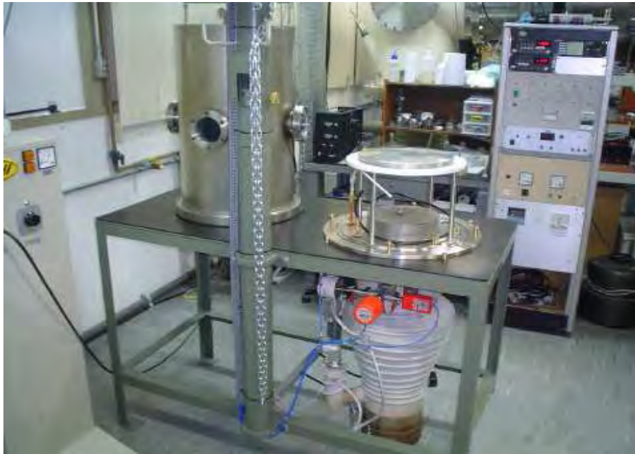
Figura 3.3 – Câmara de deposição de DLC. Fonte: Silva (2011).
