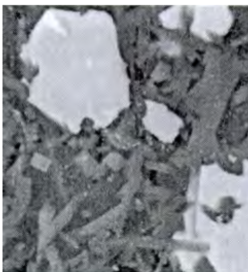
Figura 2.9 – Micrografia de BSE de basalto com uma camada condutora de ouro representando contraste dos materiais: cinza claro ( \text{Fe}_3\text{O}_4 , magnetita), cinza médio ( \text{MgFeSi}_2\text{O}_6 , piroxeno) e cinza escuro (vidro álcali-terro-álcali-aluminossilicato, em torno de 80% Si, 10% Al) Fonte: Adaptado de Reimer (1998)
