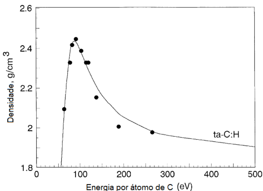
Figura 2.5 – Comparação da fração de sp^3 entre modelo e resultados laboratoriais. Fonte: Adaptado de Weiler et al (1994)
