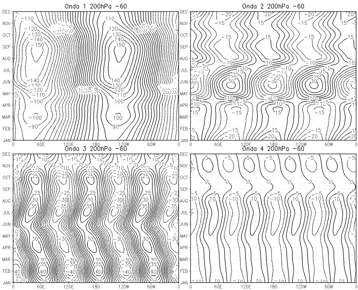
Figura 4.30 - Evolução mensal da amplitude e fase das OEs 1, 2, 3 e 4 em 60°S em 200hPa (mgp).
