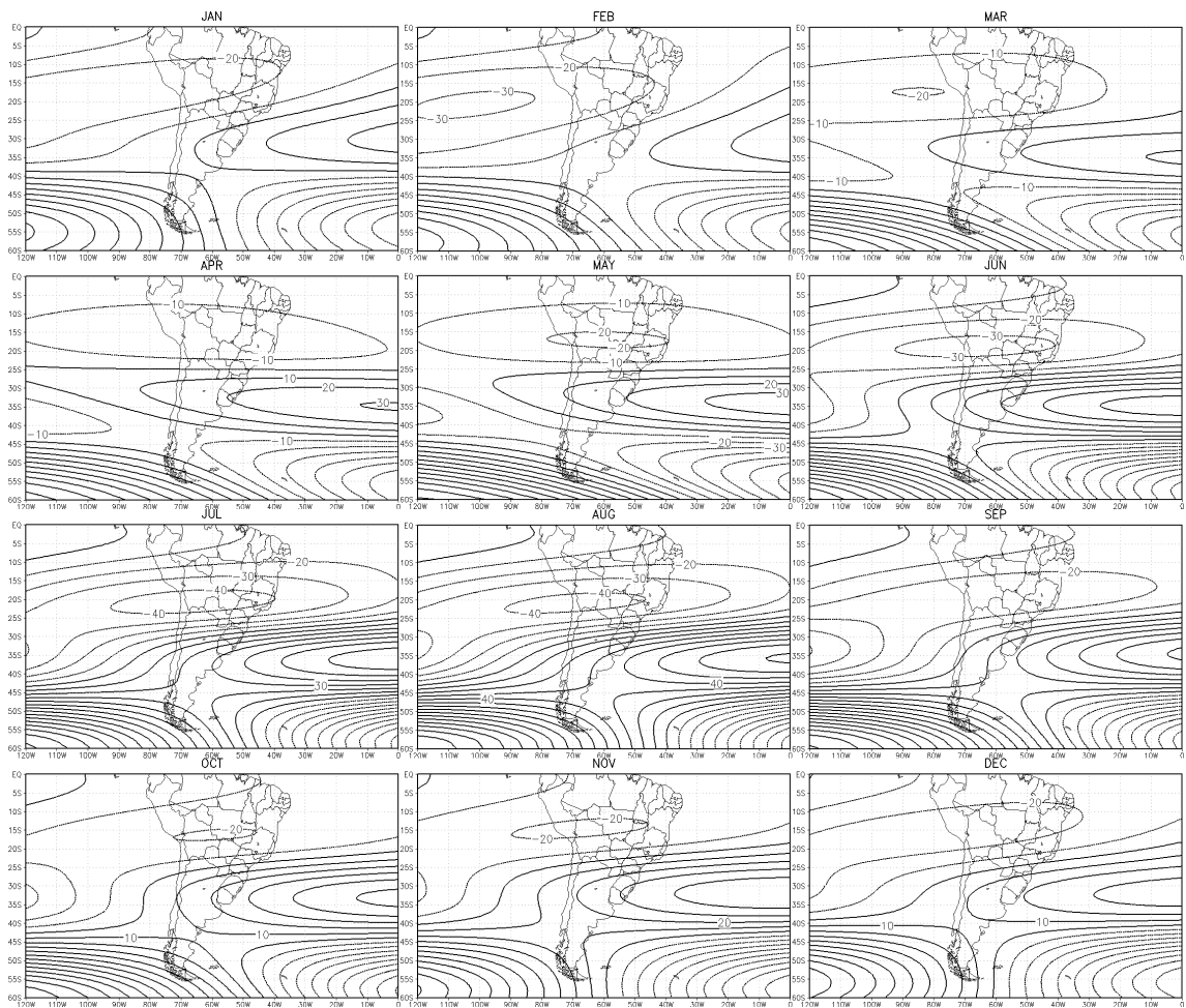
Figura 4.16 - OE 1 na AS em 200hPa (mgp).
