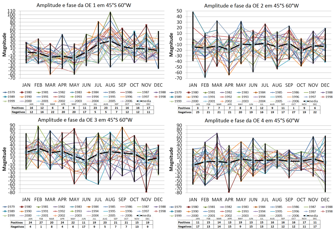
Figura 5.20 - Variabilidade da amplitude e fase das ondas 1 a 4 em 45°S, 60°W, em 200hPa (mgp), na tabela é mostrado o total de casos positivos e negativos.
