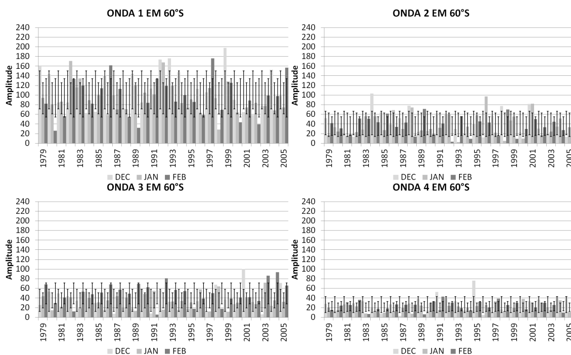
Figura 5.13 - Variabilidade interanual das amplitudes das OEs 1 a 4 em 200hPa (mgp) nos meses de dezembro, janeiro e fevereiro em 60°S, as barras indicam o desvio padrão.
