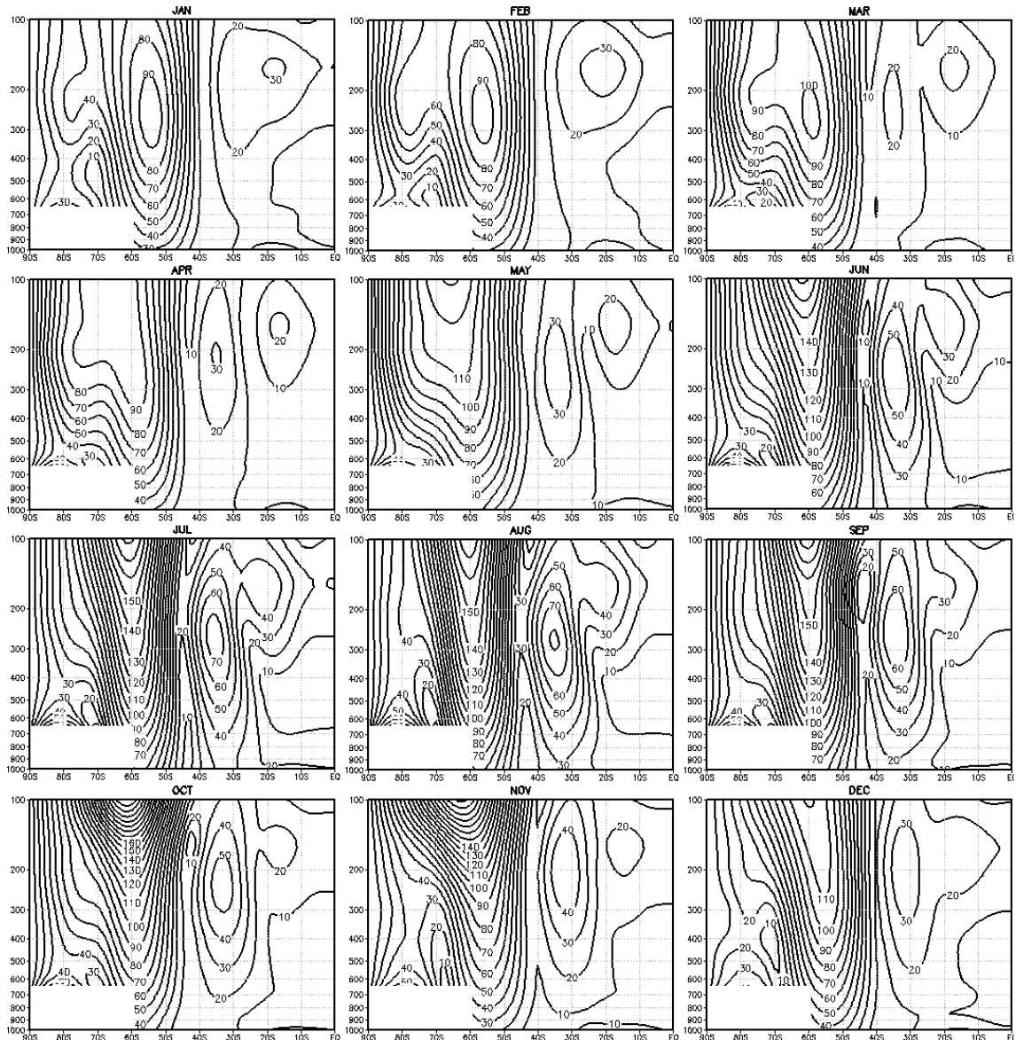
Figura 4.6 - Amplitude climatológica da OE 1 no HS (mgp).
