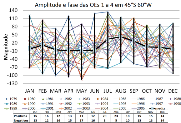
Figura 5.19 - Variabilidade da amplitude e fase somada das ondas 1 a 4 em 45°S, 60°W e 200hPa (mgp), na tabela é mostrado o total de casos positivos e negativos.
