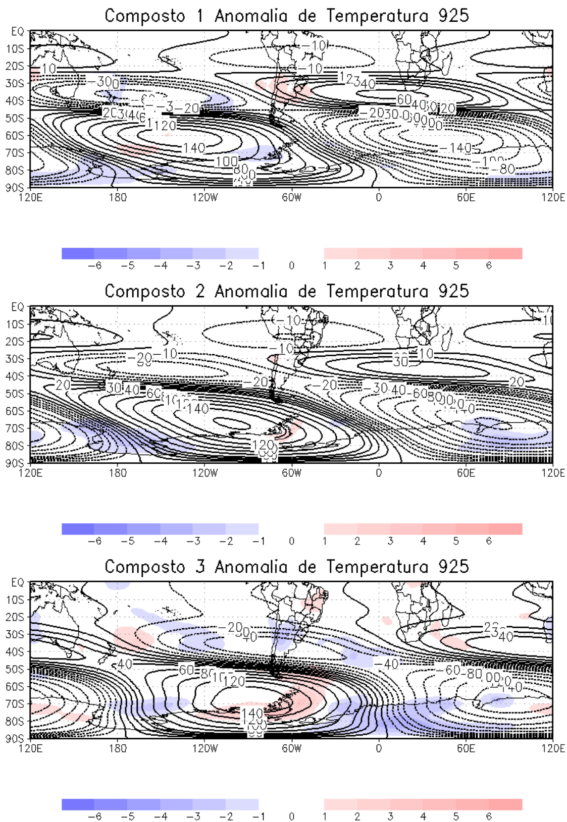
Figura 6.4 - Compostos para a OE 1 em 200hPa (mgp) para os meses de outono (linhas) e média das anomalias temperatura em 925 hPa para os meses do composto (°C), conforme Tabela 6.5.
