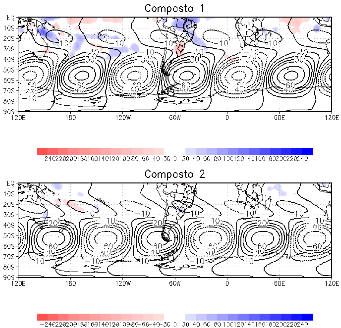
Figura 6.17 - Compostos para a OE 3 em 200hPa (mcp) para os meses de outono (linhas) e média das anomalias de precipitação para os meses do composto (mm/mês), conforme Tabela 6.7.
