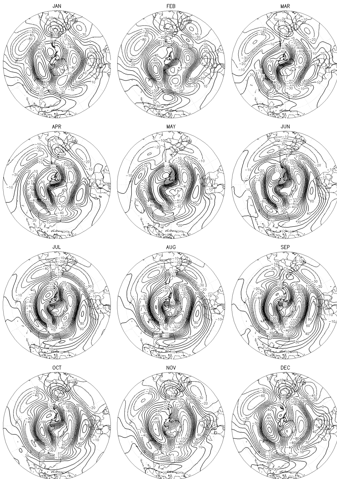
Figura 4.10 - Anomalia zonal do geopotencial em 200 hPa no HS (mgp).
