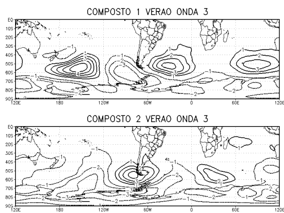
Figura A.9 - Média das anomalias mensais de PNM (hPa) para os compostos de verão da OE 3, conforme Tabela 6.7.
