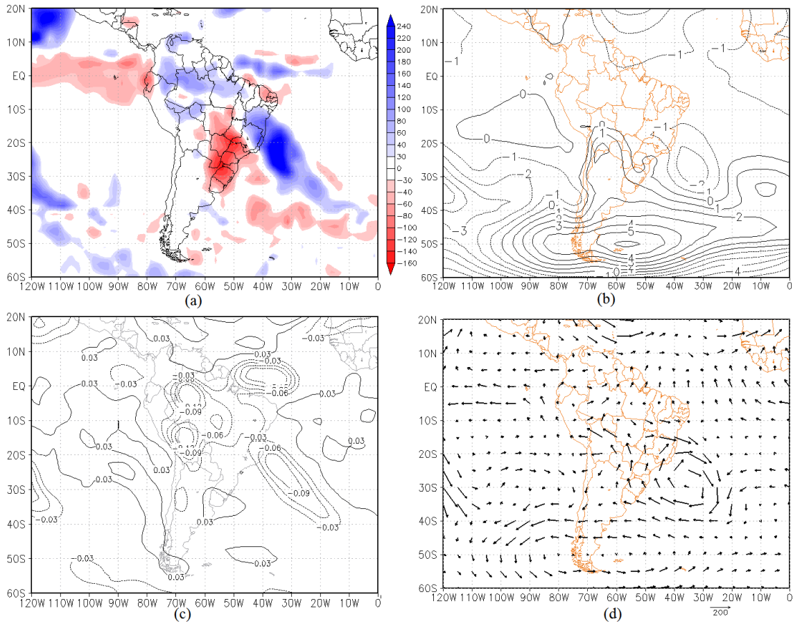
Figura 6.21 - Campos para o mês de fevereiro de 2005 (a) anomalia de precipitação (mm), (b) anomalia de pressão PNM (hPa), (c) anomalia de omega em 500 hPa (Pa/s) e (d) anomalia do fluxo de umidade integrado verticalmente (Kg/m.s).
