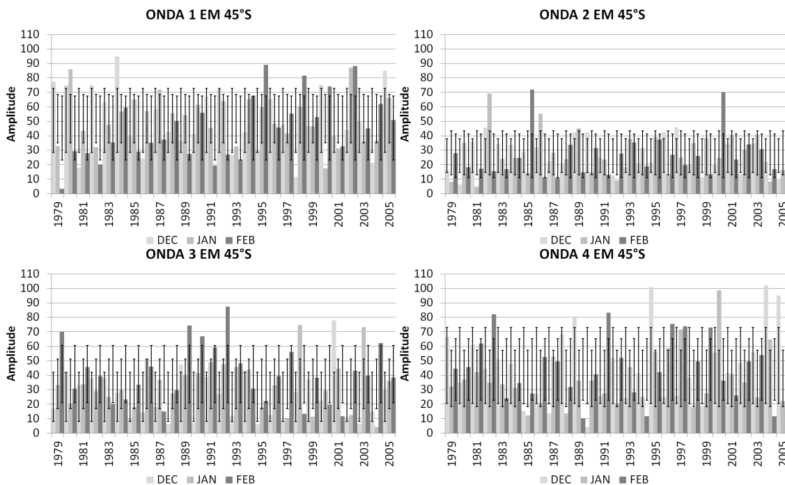
Figura 5.9 - Variabilidade interanual das amplitudes das OEs 1 a 4 em 200hPa (mgp) nos meses de dezembro, janeiro e fevereiro em 45°S, as barras indicam o desvio padrão.
