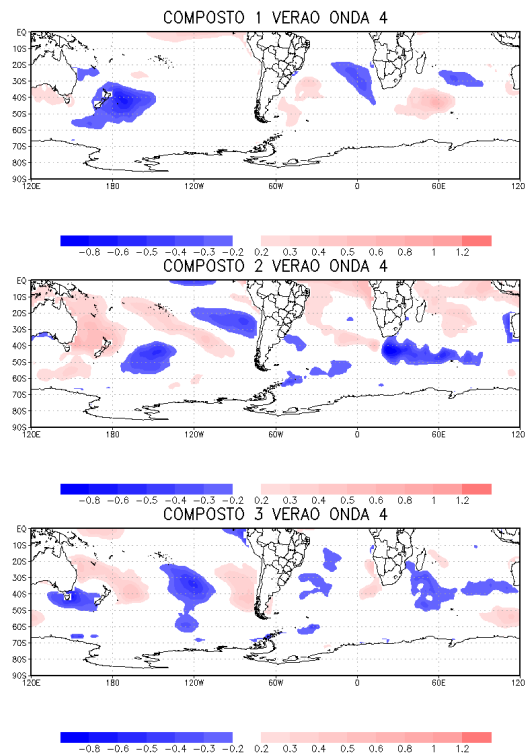
Figura A.29 - Média das anomalias mensais de TSM ( ^{\circ}\text{C} ) para os compostos de verão da OE 4, conforme Tabela 6.8.
