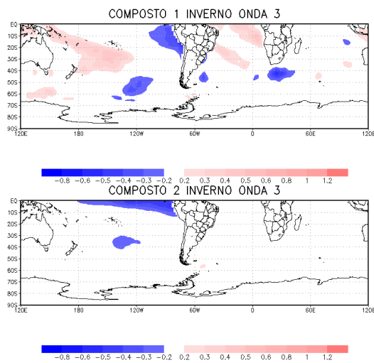
Figura A.27 - Média das anomalias mensais de TSM ( ^{\circ}\text{C} ) para os compostos de inverno da OE 3, conforme Tabela 6.7.
