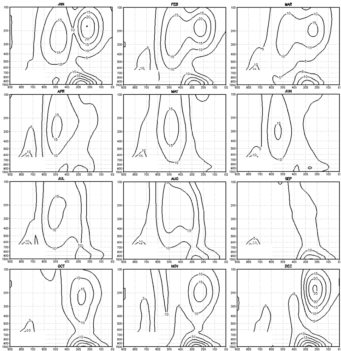
Figura 4.9 - Amplitude climatológica da OE 4 no HS (mgp).
