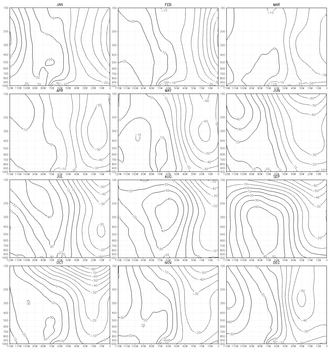
Figura 4.36 - Estrutura vertical da anomalia zonal do geopotencial em 45°S, de 0° a 120°W em 200hPa (m/g).
