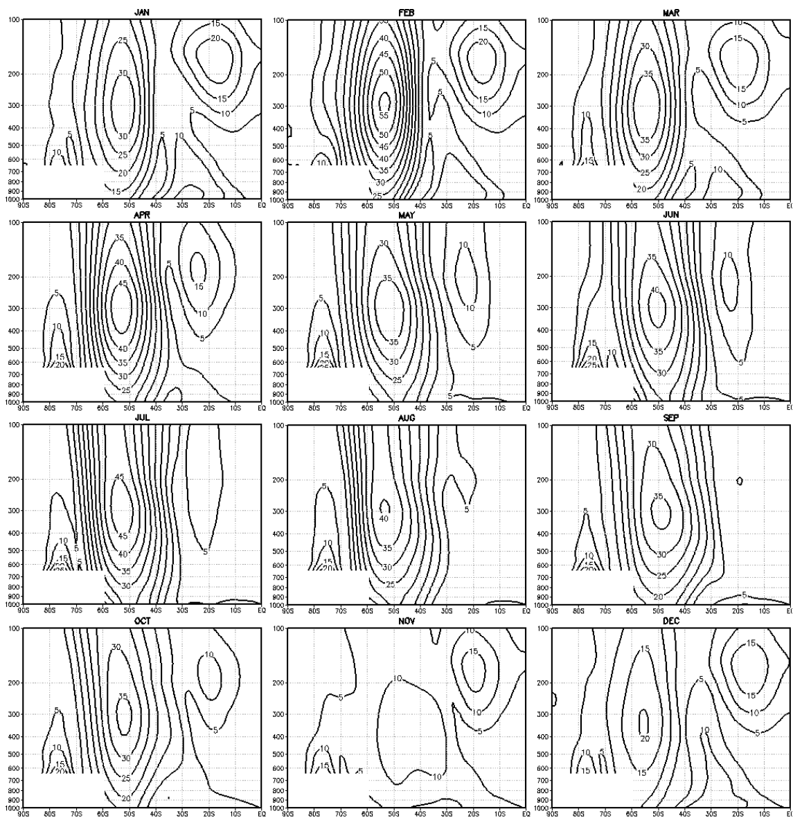
Figura 4.8 - Amplitude climatológica da OE 3 no HS (mgp).
