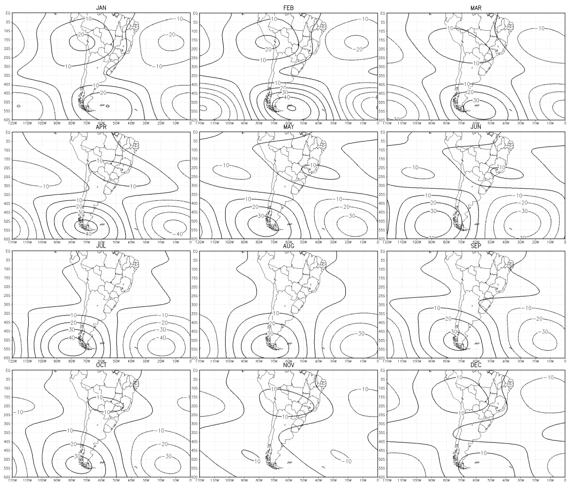
Figura 4.18 - OE 3 na AS em 200hPa (mgp).
