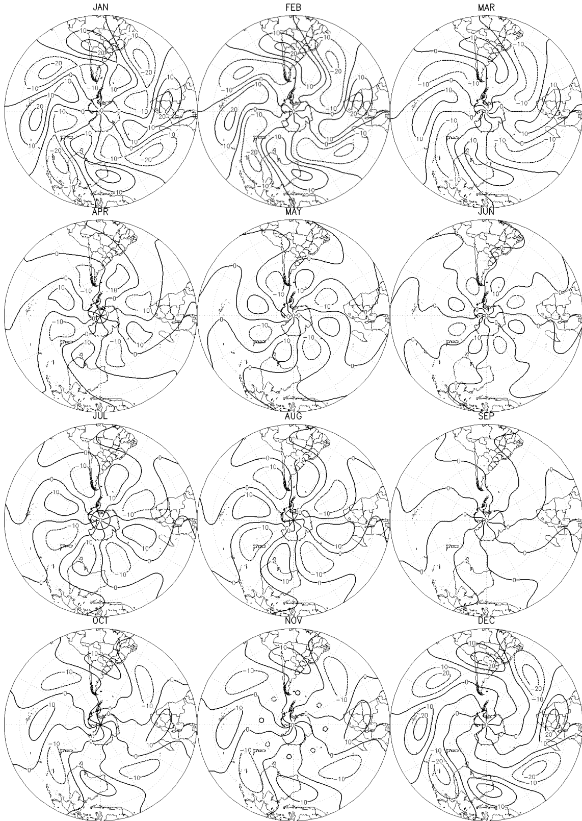
Figura 4.14 - OE 4 no HS em 200hPa (mgp).
