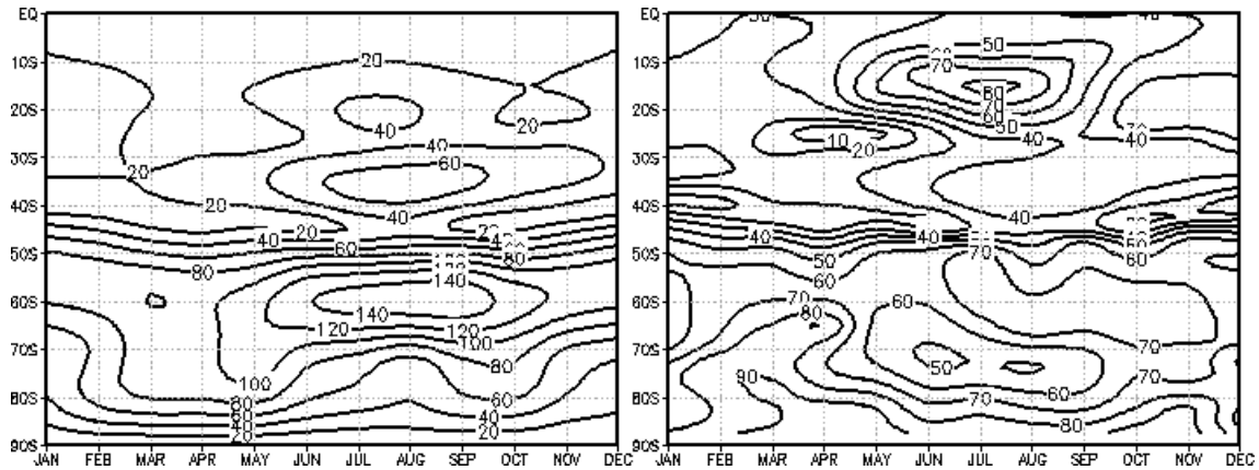
Figura 4.21 - Variabilidade mensal da Amplitude climatológica da OE 1 (mgp) no HS e a percentagem de sua representatividade relativa ao campo total.
