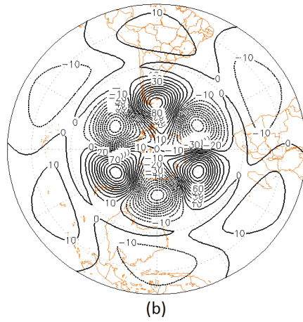
Figura 6.25 - Estrutura vertical da OE 3 em fevereiro de 2005 (a), OE 3 em 200 hPa (b) (mgp).
