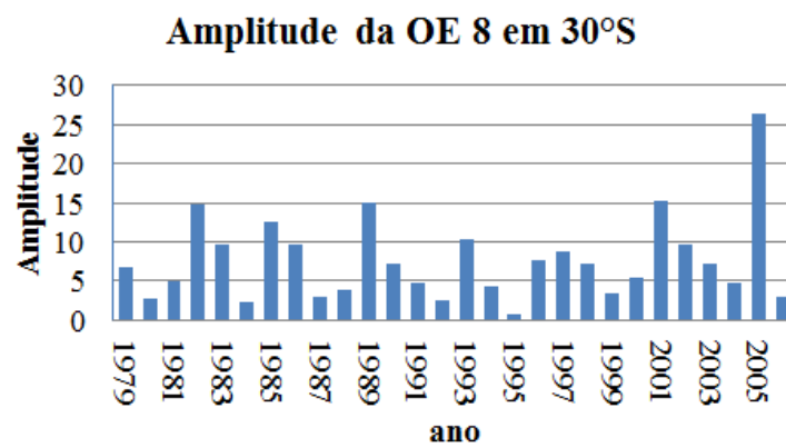
Figura 6.24 - Variabilidade interanual da amplitude (a) OE 3 em 60°S, (b) OE 6 em 3°S e (c) OE 8 em 30°S (mgp)
