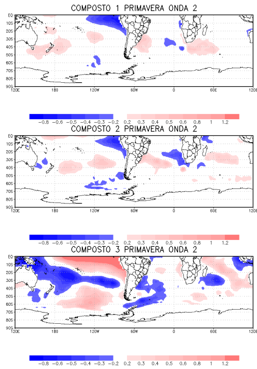
Figura A.24 - Média das anomalias mensais de TSM ( ^{\circ}\text{C} ) para os compostos de primavera da OE 2, conforme Tabela 6.6.
