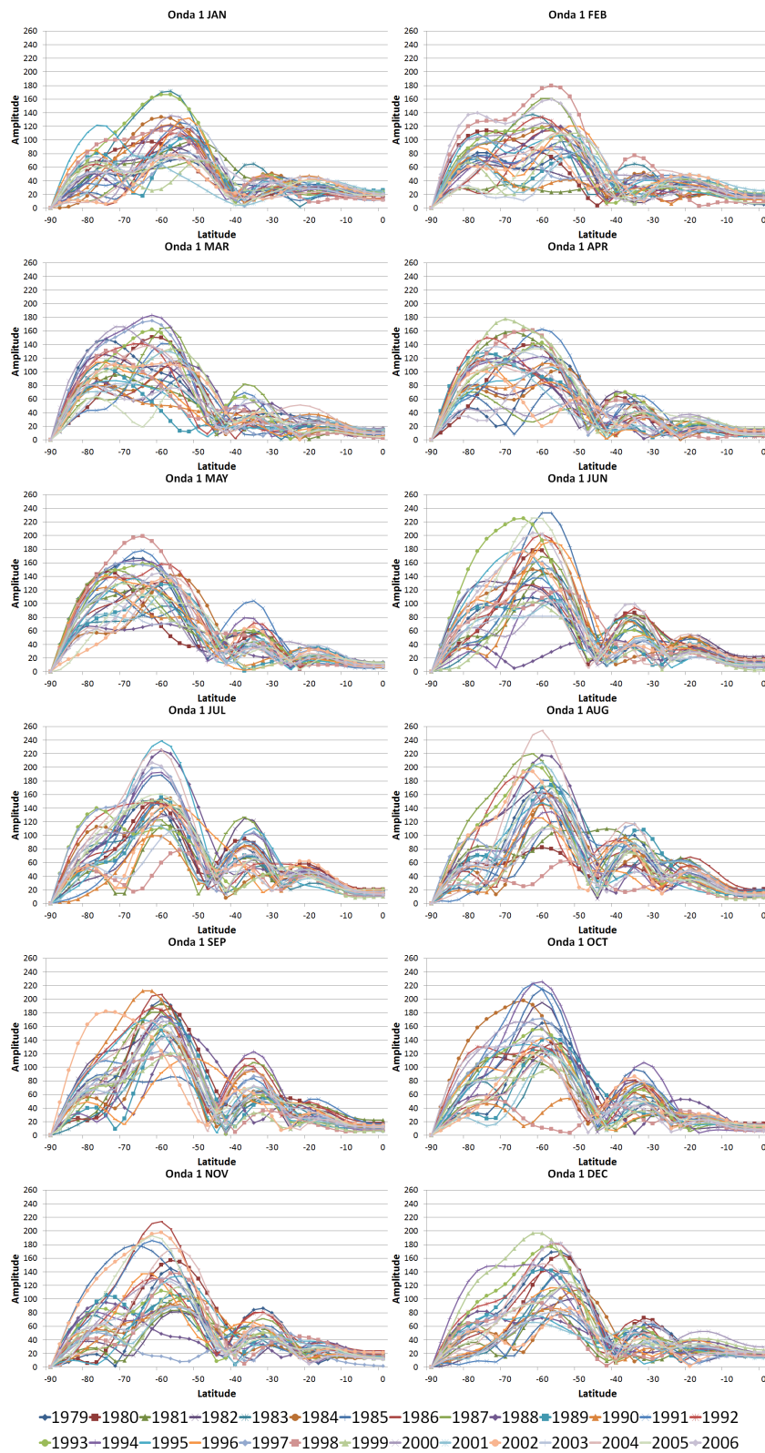
Figura 5.1 - Variabilidade interanual da amplitude da OE 1 no HS em 200 hPa (mgp).
