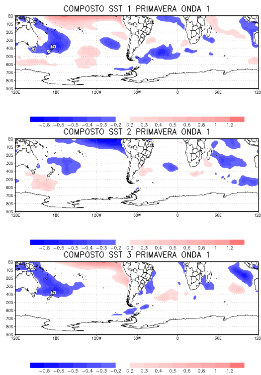
Figura A.20 - Média das anomalias mensais de TSM ( ^{\circ}\text{C} ) para os compostos de primavera da OE 1, conforme Tabela 6.5.
