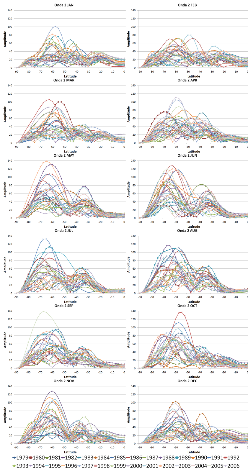
Figura 5.2 - Variabilidade interanual da amplitude da OE 2 no HS em 200 hPa (mgp).
