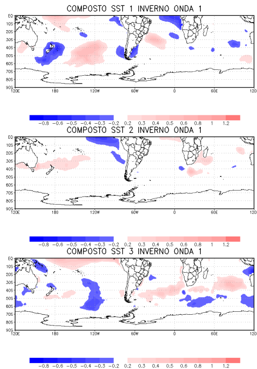
Figura A.19 - Média das anomalias mensais de TSM ( ^{\circ}\text{C} ) para os compostos de inverno da OE 1, conforme Tabela 6.5.
