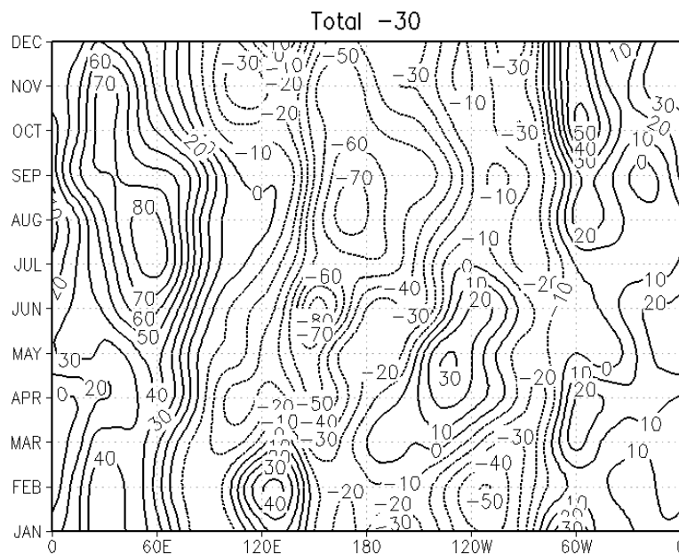
Figura 4.25 - Evolução mensal da anomalia zonal do geopotencial em 30°S em 200hPa (mgp).
