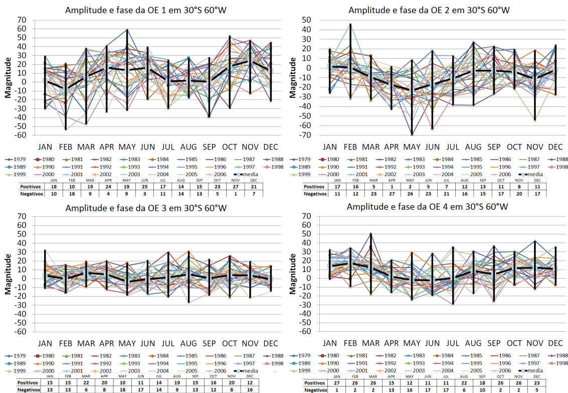
Figura 5.18 - Variabilidade da amplitude e fase das ondas 1 a 4 em 30°S, 60°W, em 200hPa (mgp), na tabela é mostrado o total de casos positivos e negativos.
