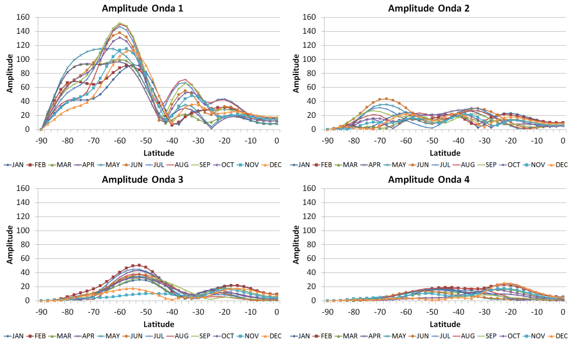
Figura 4.4 - Amplitude das ondas 1, 2, 3 e 4 em 200hPa (mgp).
