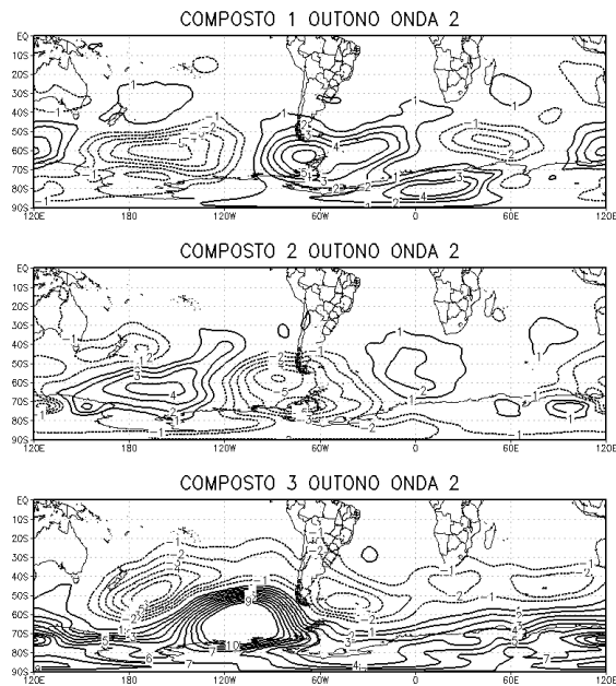
Figura A.6 - Média das anomalias mensais de PNM (hPa) para os compostos de outono da OE 2, conforme Tabela 6.6.
