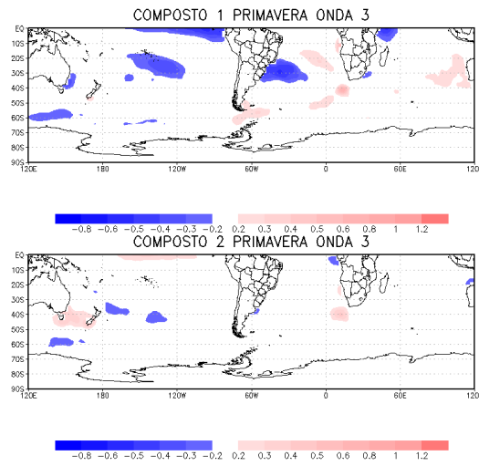
Figura A.28 - Média das anomalias mensais de TSM ( ^{\circ}\text{C} ) para os compostos de primavera da OE 3, conforme Tabela 6.7.
