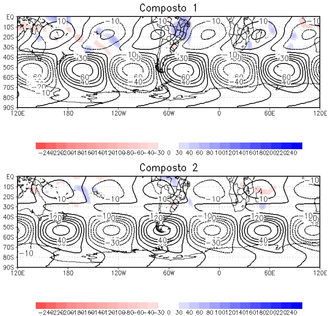
Figura 6.16 - Compostos para a OE 3 em 200hPa (mgp) para os meses de verão (linhas) e média das anomalias de precipitação para os meses do composto (mm/mês), conforme Tabela 6.7.
