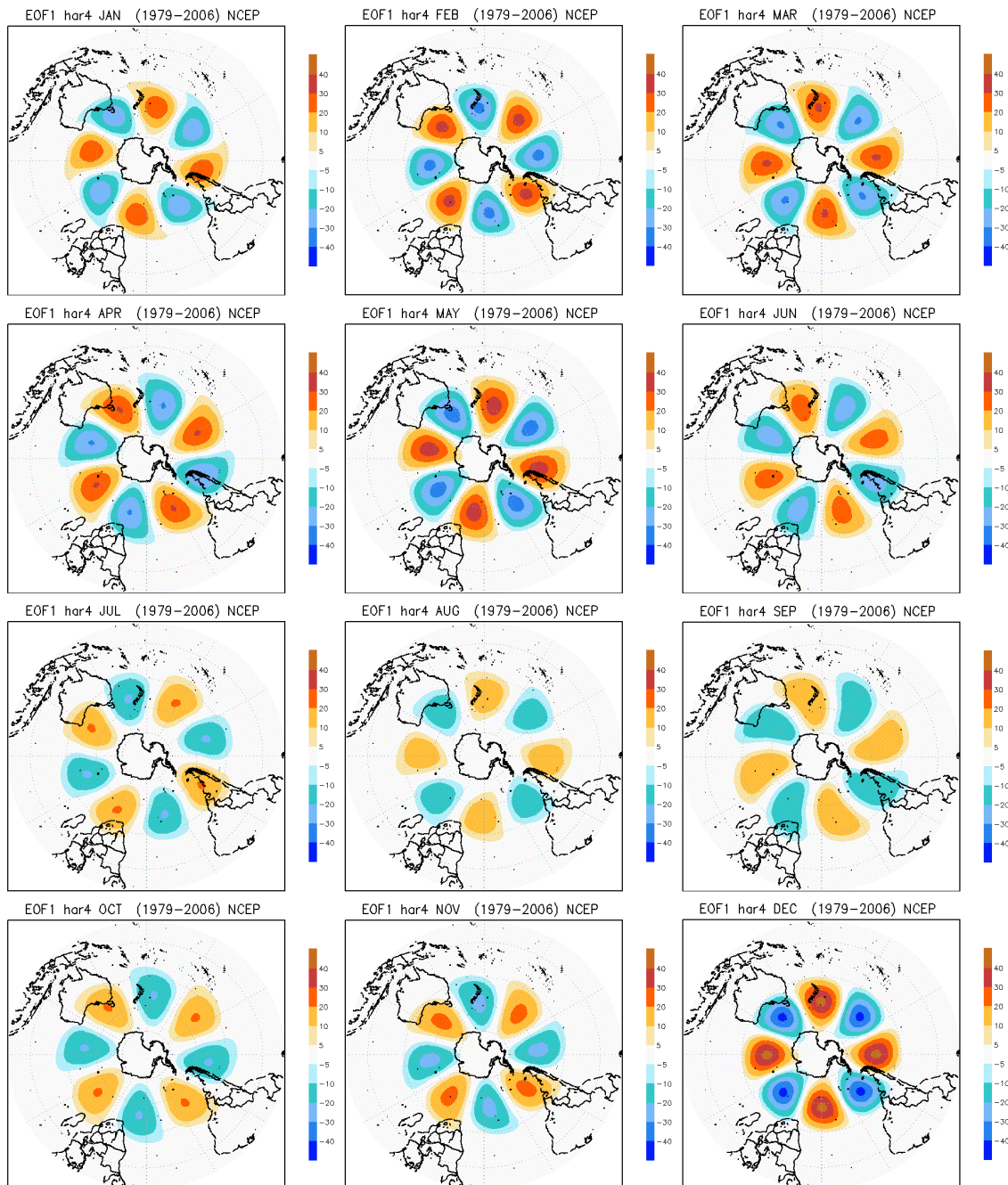
Figura 5.26 - Modo dominante de variabilidade da onda 4 nos 12 meses do ano.
