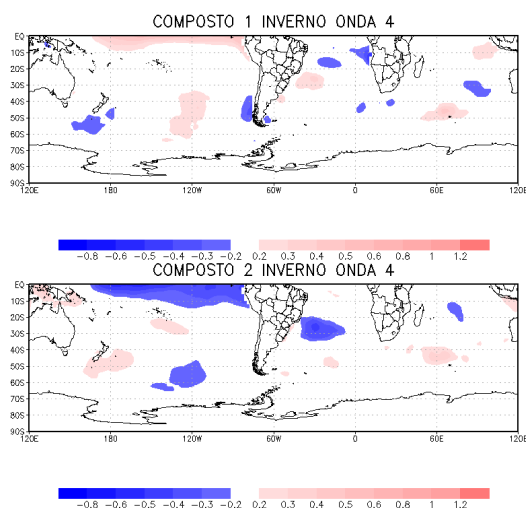
Figura A.31 - Média das anomalias mensais de TSM ( ^{\circ}\text{C} ) para os compostos de inverno da OE 4, conforme Tabela 6.8.
