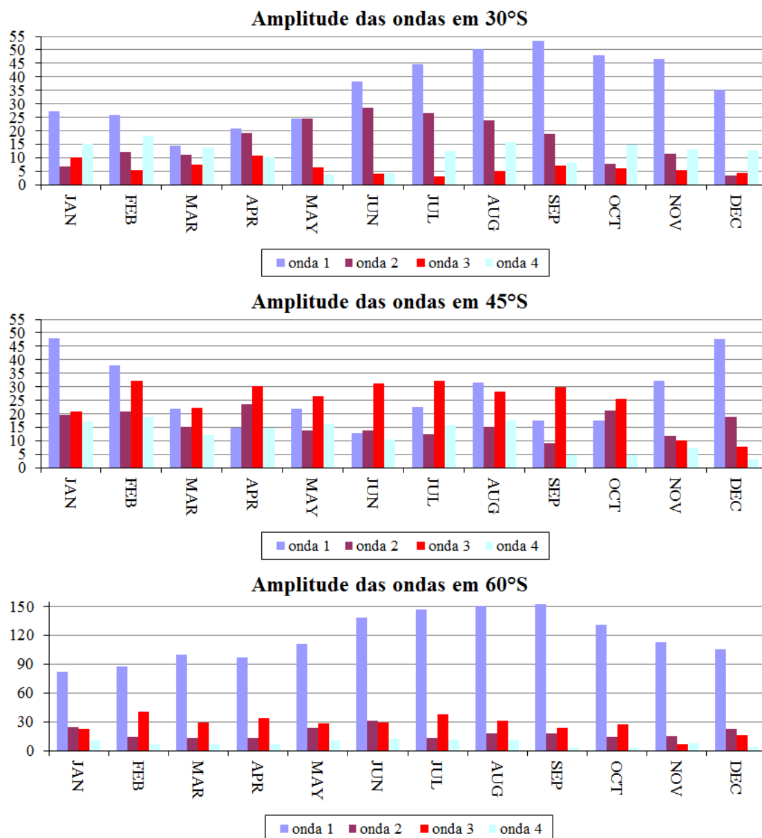
Figura 4.1 - Amplitude das 4 principais OE em 30°S, 45°S e 60°S, em 200 hPa (mgp).
