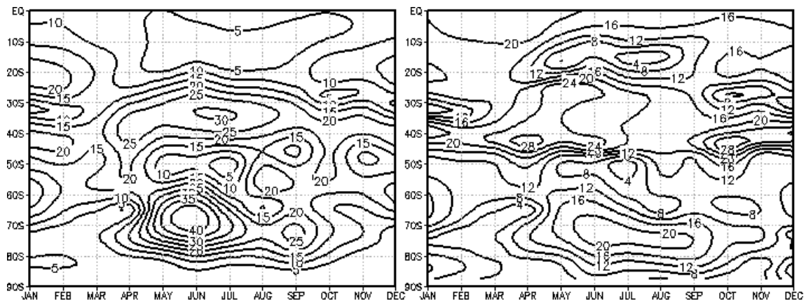
Figura 4.22 - Variabilidade mensal da Amplitude climatológica da OE 2 (mgp) no HS e a percentagem de sua representatividade relativa ao campo total.
