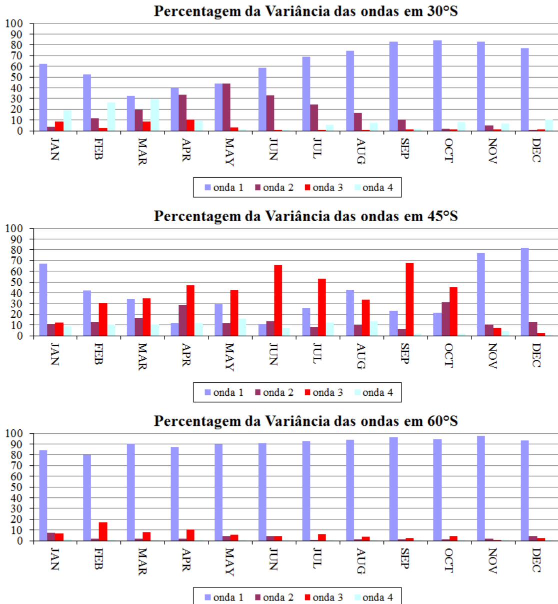
Figura 4.2 - Percentagem da variância das 4 principais OE em 30°S, 45°S e 60°S em 200 hPa.
