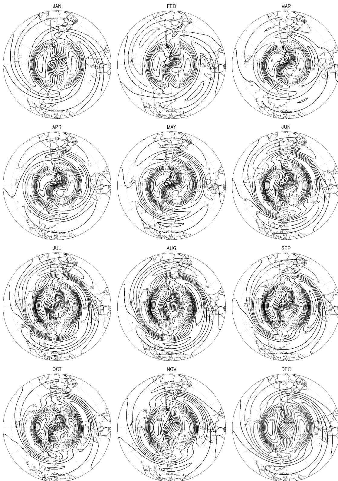
Figura 4.11 - OE 1 no HS em 200hPa (mgp).
