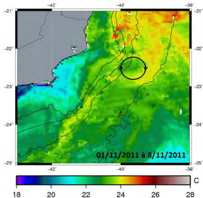
Figura 4.19 – TSM média de 8 dias (01/11 a 08/11/2011), estimada com dados MODIS Aqua , resolução de 4 km. O campo de TSM indica o vórtice ciclônico, centrado em 22°30'S-39°30'W, com temperatura superficial de 24°C em seu entorno e um núcleo relativamente mais frio (23°C).
