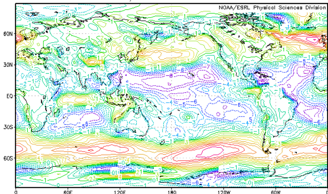
Figura 3.3 – Campo de vento meridional à 10 m acima da superfície, média mensal em dezembro de 2011. Fonte: NCEP Reanalysis data obtido pela NOAA/OAR/ESRL PSD, Boulder, Colorado, USA, pelo site http://www.esrl.noaa.gov/psd/ .
