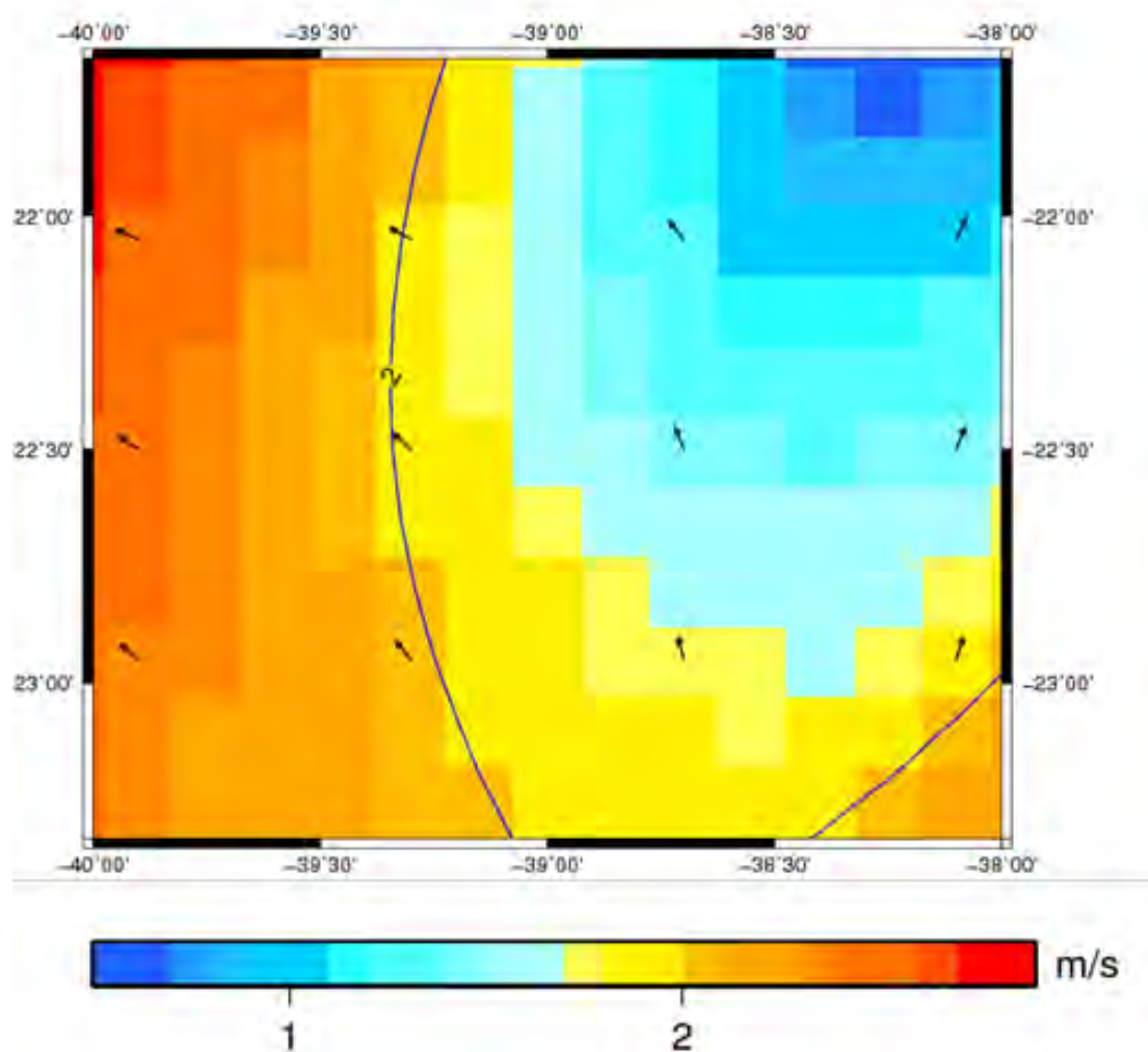
Figura 4.23 - Campo de vento na superfície do mar, obtido da reanálise NCEP em 12/11/2011 18:00 GMT. A isolinha da magnitude de 2 m/s coincide com a inversão no contraste óleo-água na pluma próxima ao foco do vazamento.
