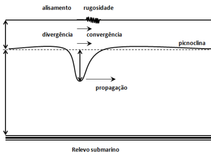
Figura 4.34 - Visão esquemática da onda interna solitária formando zonas de convergência acima da termoclina (ou picnoclina) que resultam em modulações da rugosidade na superfície marinha, (Fonte: adaptada de ROBINSON, 2004).
