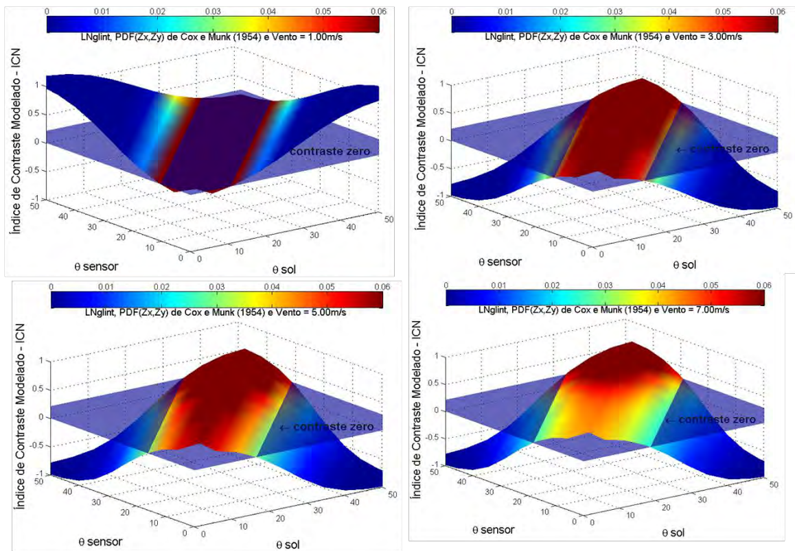
Figura 3.5 – Contraste modelado pelo ICN em diferentes condições geométricas de aquisição por sensor remoto e diferentes magnitudes do vento.
