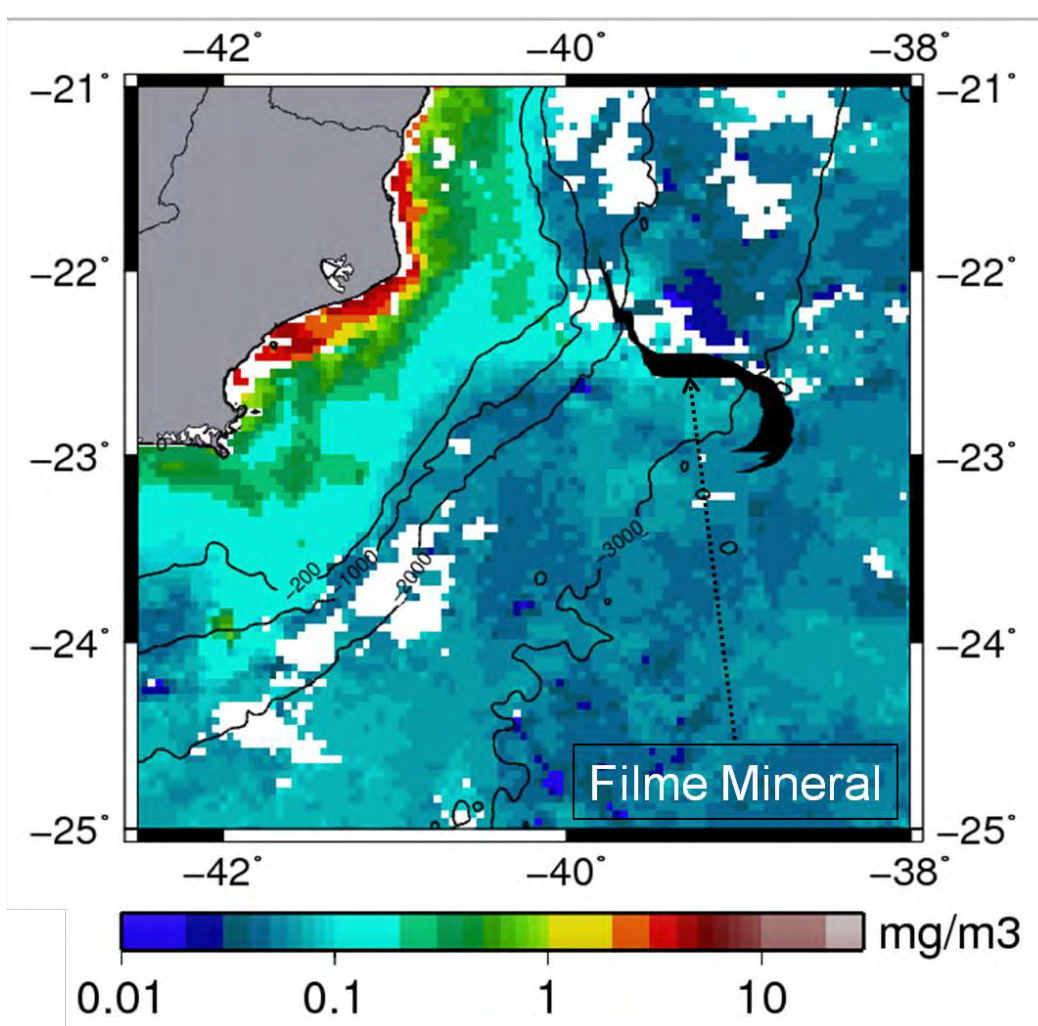
Figura 4.17 - Concentração de clorofila média do mês de novembro de 2011, estimada pelo sensor MODIS Aqua , com resolução de 4 km. Pode-se observar baixos valores na área de ocorrência do filme mineral.
