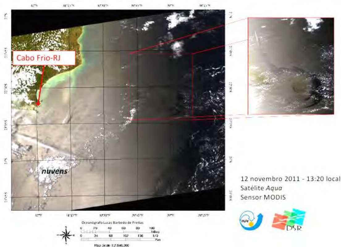
Figura 4.15- Vazamento de óleo na Bacia de Campos, observado em imagem MODIS Aqua de 12/11/2011 16:20 GMT, em condições de sunglint . A geometria de aquisição (sol e sensor) e a rugosidade superficial, imposta pelo vento, resultam em uma ampla faixa de alta reflexão especular bidirecional na superfície do oceano.
