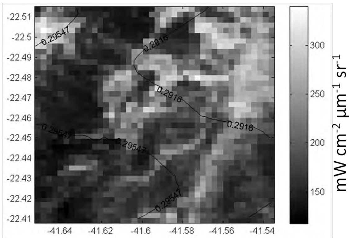
Figura 4.12 – Superfície com biofilme 26/01/2003 às 13:35 GMT: radiâncias TOA geolocalizadas e calibradas, MODIS nível 1B, banda 645 nm, em condição de sunglint. Isolinhas de contorno representam o índice de contraste normalizado – ICN (ver texto). As áreas de radiâncias mais intensas são atribuídas à presença de biofilmes originais de Trichodesmium .
