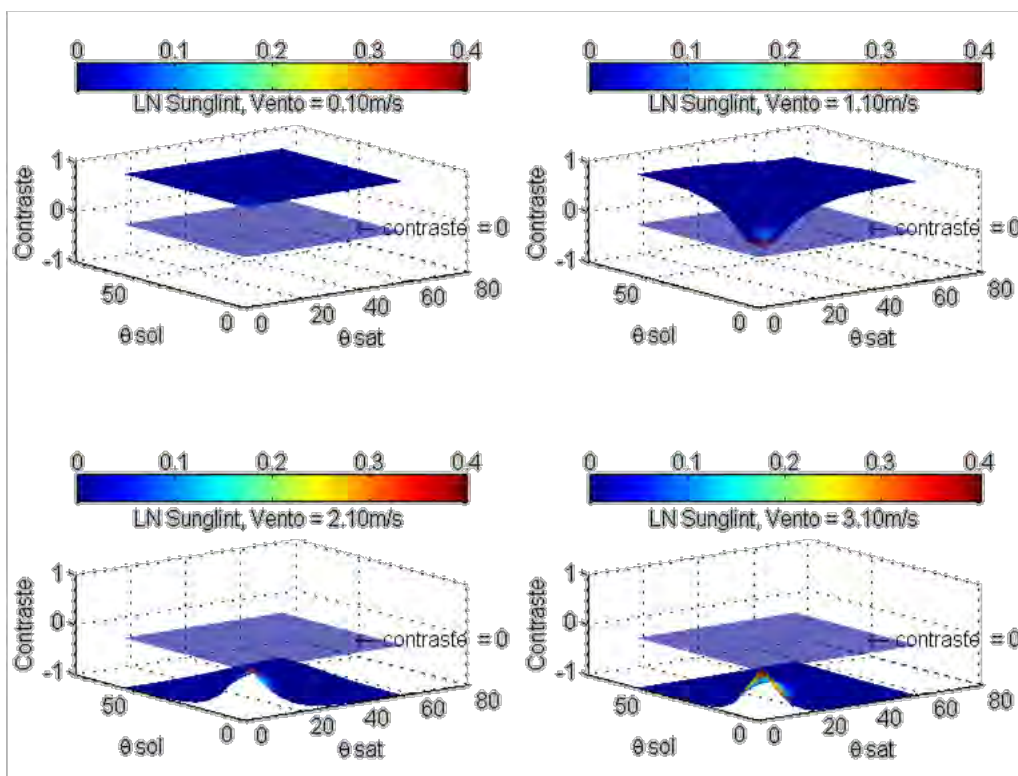
Figura 4.25 - Característica do LN_{glint} e contraste do filme surfactante em relação a áreas limpas vizinhas avaliado pelo ICN, para geometria de aquisição (sol/sensor) de zênite similar à aquisição MODIS de 12/11/2012 16:20 GMT, com azimuth relativo -157^\circ e vento entre 0-3 m/s.
