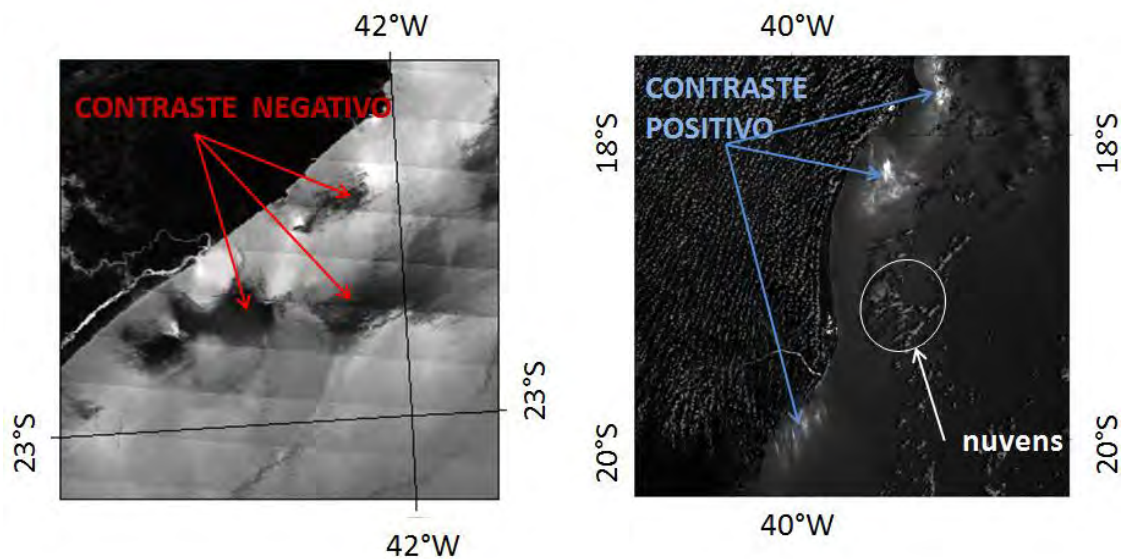
Figura 3.4 - Contraste negativo em filmes superficiais em imagem MODIS Terra de 3/02/2010 na banda centrada em 645 nm (Esquerda). Contraste positivo em filmes superficiais em imagem MODIS Aqua de 22/01/2010 (Direita). Feições têm origem provável de agentes surfactantes de origem continental por aporte de rios e da alta produção biológica costeira. Outros agentes também causam variações no campo de sunlint como variações no vento, na dinâmica superficial marinha e contaminação por nuvens.
