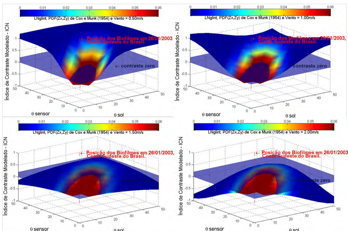
Figura 4.10 - Contraste modelado na superfície do mar para a presença de biofilmes avaliada pelo ICN. As condições geométricas de aquisição via sensoriamento remoto e ventos na superfície do mar são idênticas as da aquisição de imagens do MODIS Terra em 26/01/2003 13:35 GMT. As condições geométricas de aquisição na área de influência dos biofilmes são \varphi_v - \varphi_s = -161^\circ , \varphi_v = 18.5^\circ e \varphi_s = 24^\circ .
