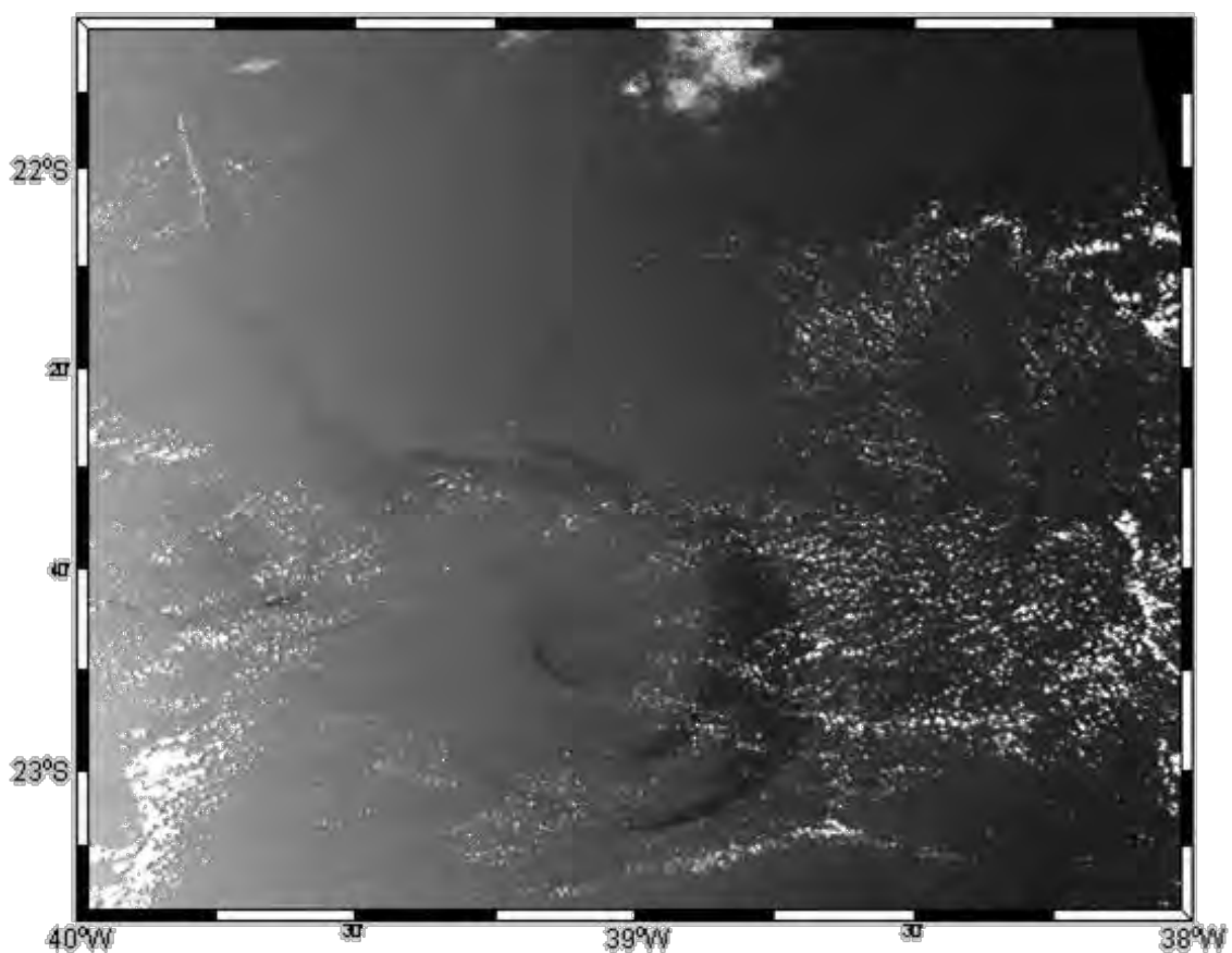
Figura 4.22 - Imagem MODIS 12/11/2011 16:20GMT, banda 645 nm, resolução espacial 250 m, destacando a feição de óleo oriunda do vazamento no Campo de Frade, Bacia de Campos, RJ.
