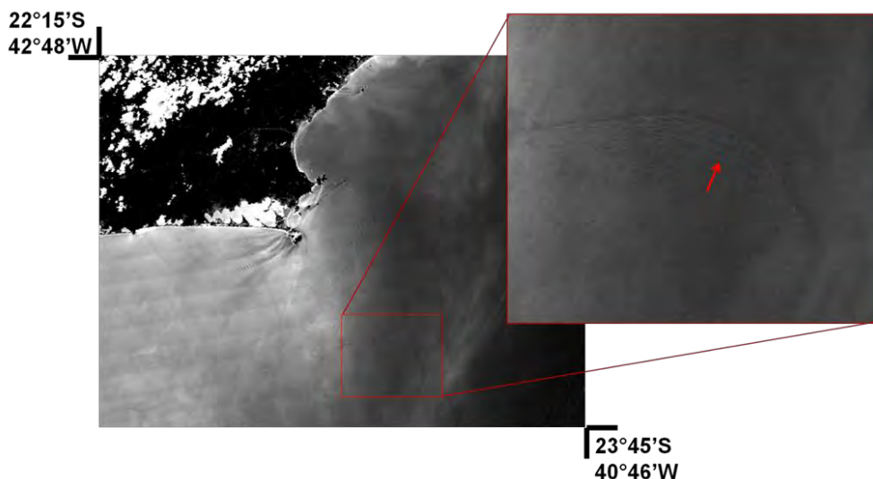
Figura 4.33 – MODIS Aqua de 06/11/2009 16:25 GMT, resolução 250m. Onda interna solitária com radiais concêntricas alternando regiões brilhantes e escuras, destacada pela ampliação e seta vermelha.
