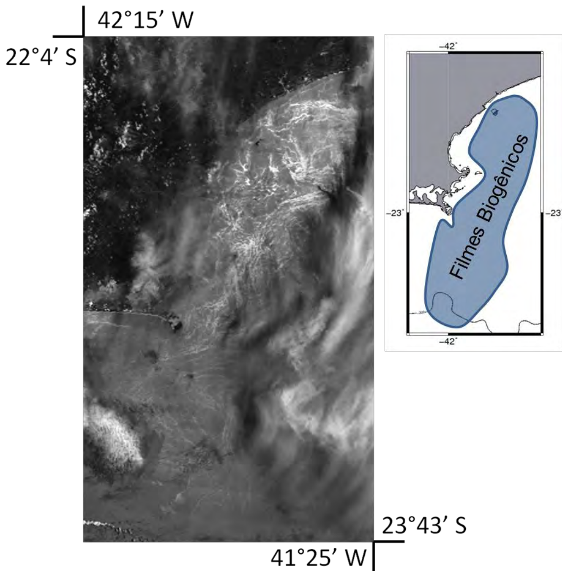
Figura 4.7 - Imagem MODIS Terra , resolução 250 m, nível L1B em condição de sun glint na banda 469 nm de 26/01/2003 às 13:35 GMT, indica com contraste positivo a presença de filmes biogênicos associados à bloom fitoplanctônico.
