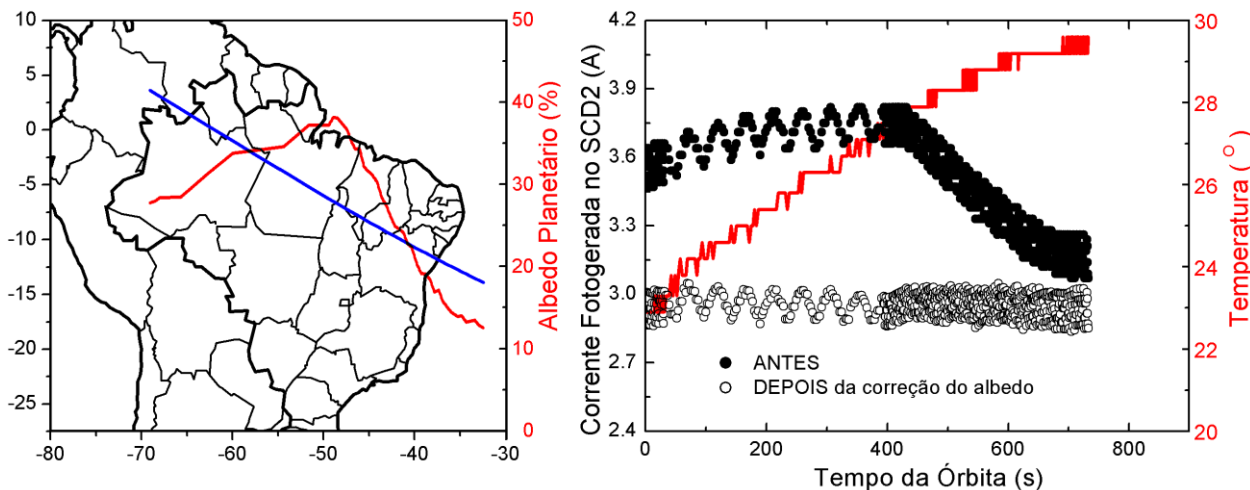
Figura 6- Curvas da órbita, do albedo, da temperatura e dados de correntes fotogeradas tomados em 01/01/2004.
