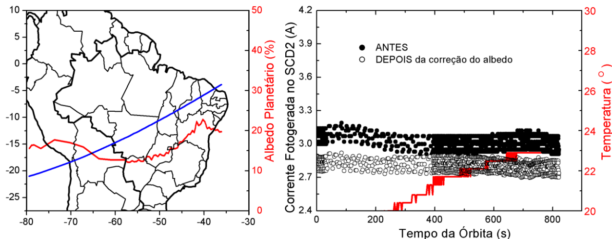
Figura 5- Curvas da órbita, do albedo, da temperatura e dados de correntes fotogeradas tomados em 01/07/2003.
