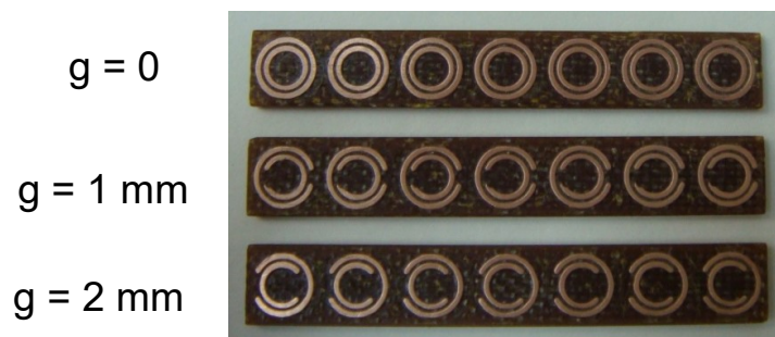
Figura 3. Diferentes redes de anéis concêntricos: com aberturas de g = 1 mm, g = 2 mm e anéis fechados ( g = 0 ).
