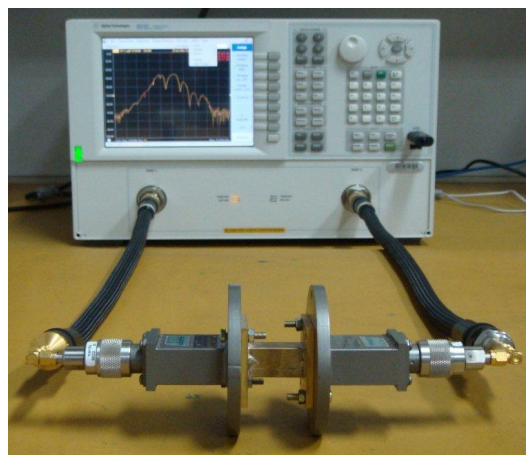
Figura 5. Montagem experimental completa conectada ao analisador de rede para medir o espectro de transmissão das redes de ressonadores de anéis concêntricos.
