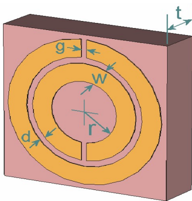
Figura 1. Ressonador de anéis repartidos.
