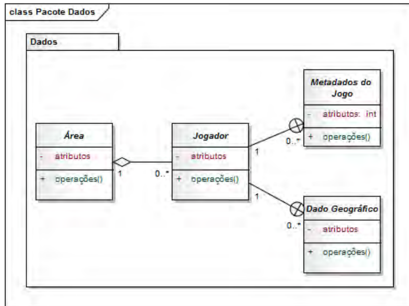
Figura 3.5 - Diagrama de classes abstratas do pacote Dados .
