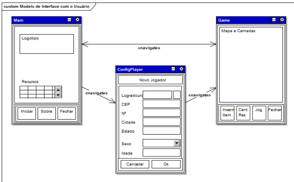
Figura 4.7 - Diagrama do modelo de interface com o usuário.
