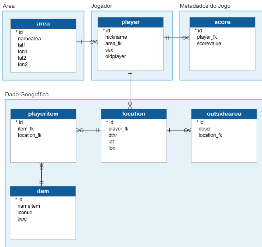
Figura 4.12 - Diagrama entidade-relacionamento das tabelas gerenciadas pelo SGBD .
