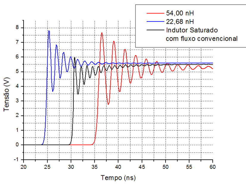
Figura 5.6 - Comparação dos pulsos saída entre linha híbrida com indutor saturado de fluxo convencional e LTNLs com indutores fixos e sem perdas.
