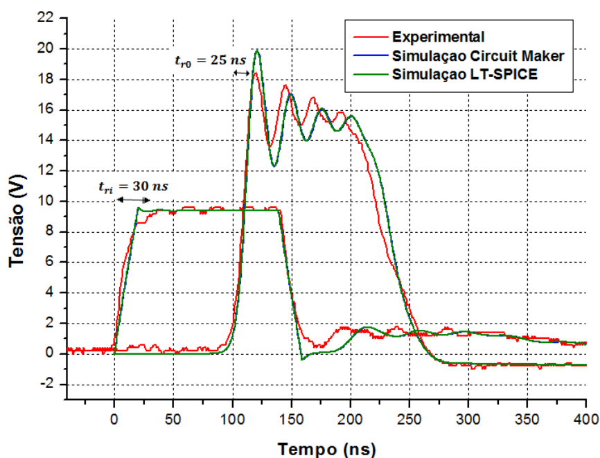
Figura 5.5 - Comparação de resultados para os pulsos de entrada (pulso quadrado) e saída (pulso oscilatório) no caso oscilatório.
