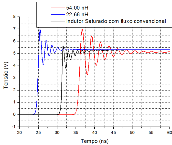
Figura 5.10 - Comparação com perdas dos pulsos de saídas de LTNLs com indutores fixos e linha híbrida com indutor saturado de fluxo convencional.
