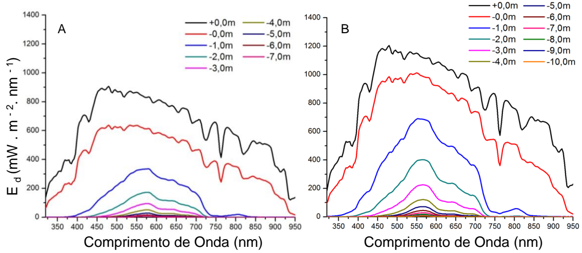
Figura A. 55: Irradiância descendente para o ponto 29 em: (A) Maio; (B) Setembro.
