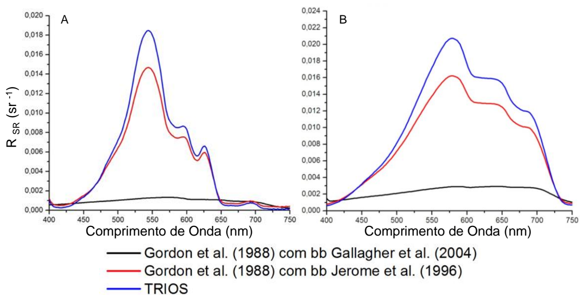
Figura B. 1: Modelos ópticos para o ponto 03 em: (A) Maio; (B) Setembro.
