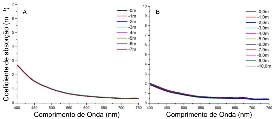
Figura A. 58: Coeficiente de absorção para o ponto 29 em: (A) Maio; (B) Setembro.
