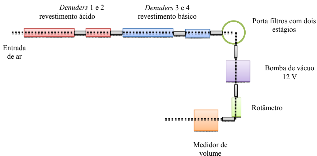
Figura 2.1 - Esquema da sequência de dispositivos utilizado no sistema SAAD (adaptado de Sutton et al., 2001).
