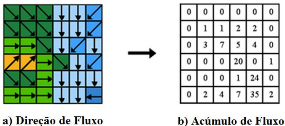
Figura 3.10 - Fluxo acumulado em cada célula de um modelo digital de elevação. Fonte: ESRI (2010).
