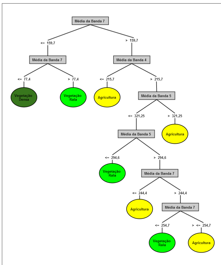
Figura 4.2 - Árvore de decisão gerada através do algoritmo j48 para classificar a imagem do período de 1984.
