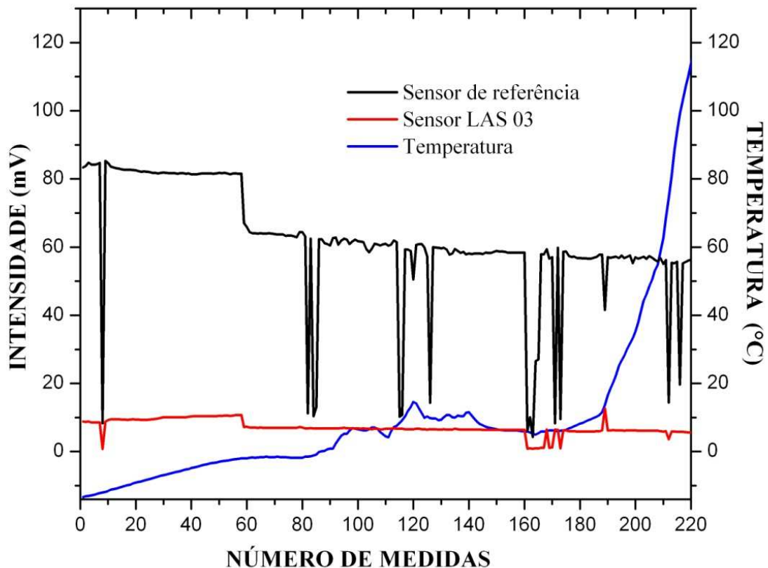
Figura 59 - Efeito da temperatura medida ao ar livre.
