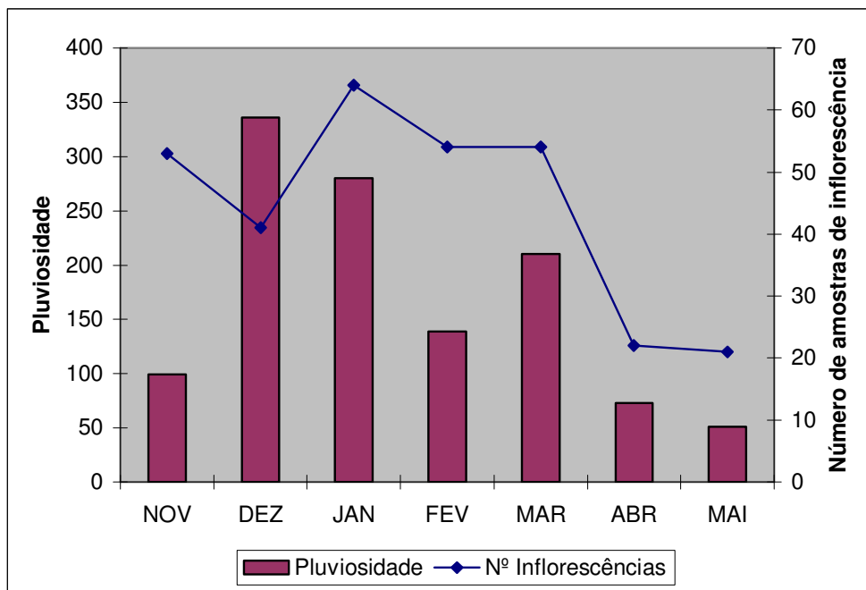
FIGURA 8: Relação entre pluviosidade e quantidade de amostras coletadas em São José dos Campos entre novembro de 2009 e junho de 2010.
