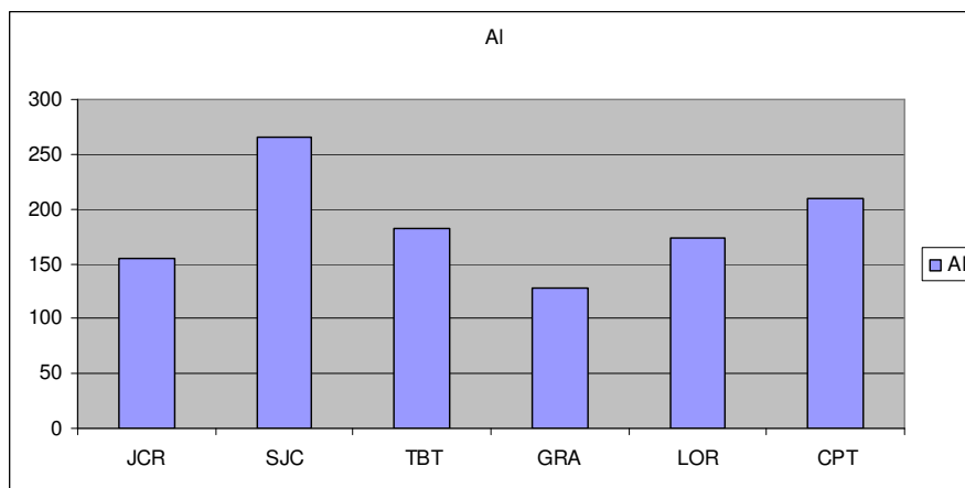
FIGURA 12 Valores médios de concentração ( \mu\text{g.g}^{-1} ), de Cl, K e Al para os 6 Municípios do Vale do Paraíba, referentes à coleta de folhas de Tradescantia pallida , após exposição de novembro de 2009 a março de 2010.
