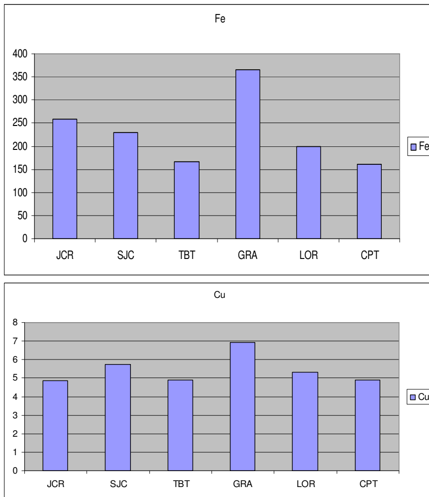
FIGURA 9 - Valores médios de concentração ( \mu\text{g}\cdot\text{g}^{-1} ), de Mn, Fe e Cu para os 6 Municípios do Vale do Paraíba, referentes à coleta de folhas de Tradescantia pallida , após exposição de novembro de 2009 a março de 2010.
