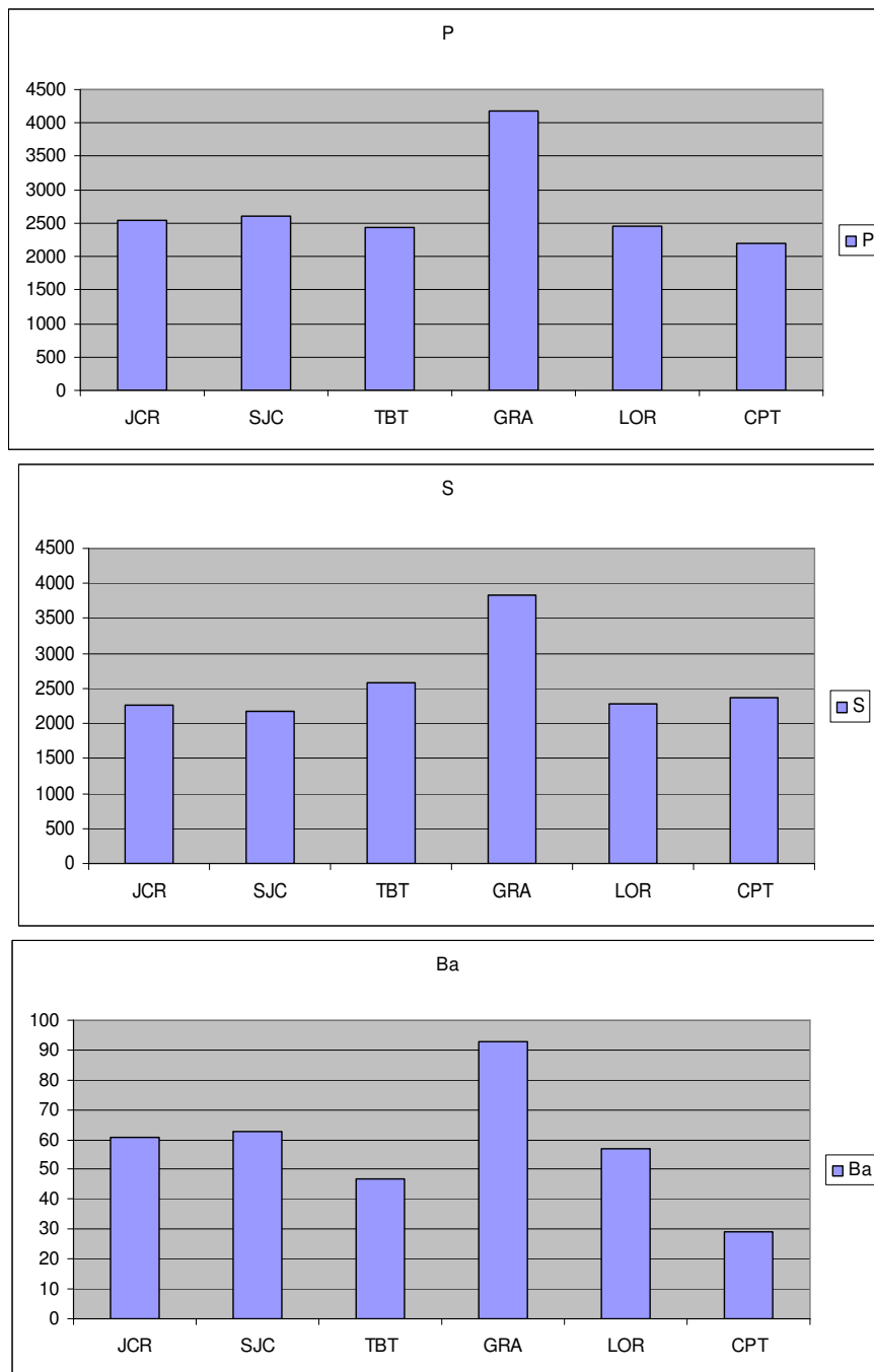
FIGURA 11 Valores médios de concentração ( \mu\text{g.g}^{-1} ), de P, S e Ba para os 6 Municípios do Vale do Paraíba, referentes à coleta de folhas de Tradescantia pallida , após exposição de novembro de 2009 a março de 2010.
