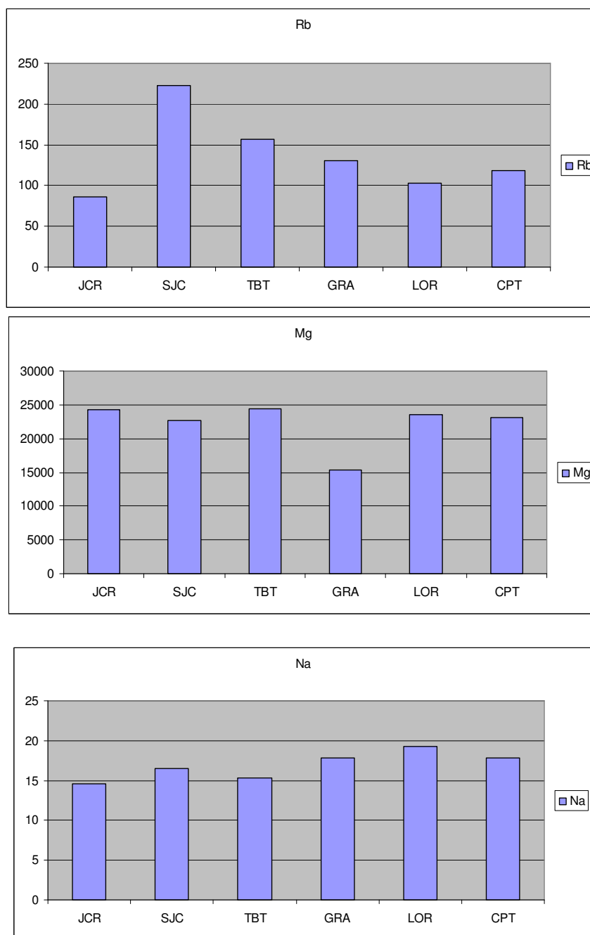
FIGURA 13 Valores médios de concentração ( \mu\text{g.g}^{-1} ), de Rb, Mg e Na para os 6 Municípios do Vale do Paraíba, referentes à coleta de folhas de Tradescantia pallida , após exposição de novembro de 2009 a março de 2010.
