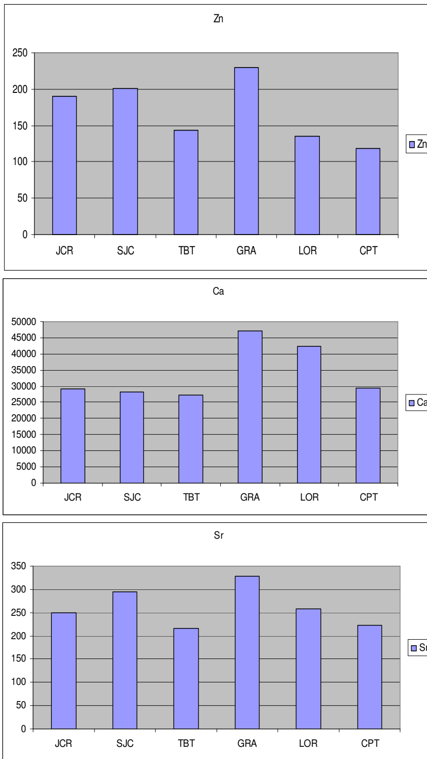
FIGURA 10- Valores médios de concentração ( \mu\text{g.g}^{-1} ), de Zn, Ca e Sr, para os 6 Municípios do Vale do Paraíba, referentes à coleta de folhas de Tradescantia pallida , após exposição de novembro de 2009 a março de 2010.
