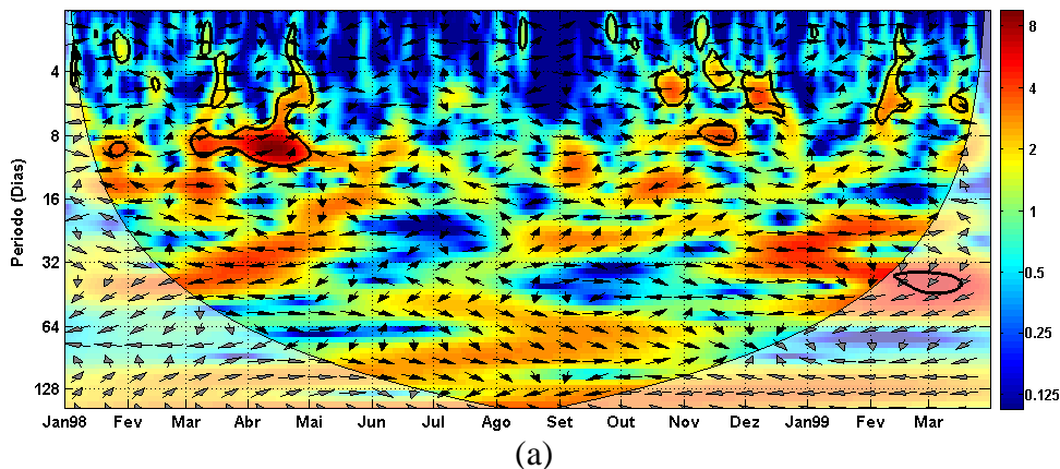
(a) Figura 4.11 - Como na Fig. 4.7, mas para ondeleta cruzada entre a AROLE não-filtrada em um ponto no sul da Austrália e a AROLE não-filtrada em um ponto na área sul da ZCAS. (Continua).
