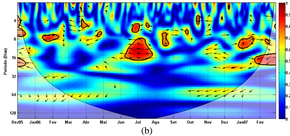
Figura 4.32 - Como na Fig. 4.7, mas para ondeleta cruzada entre a AROLE não-filtrada em um ponto no centro-leste do Pacífico sul subtropical e a AROLE não-filtrada em um ponto na área central da ZCAS.
