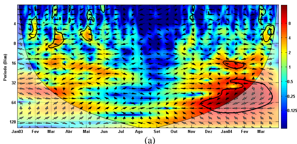
Figura 4.47 - Como na Fig. 4.7, mas para ondeleta cruzada entre a AROLE não-filtrada em um ponto no oeste do Pacífico sul tropical e a AROLE não-filtrada em um ponto na área norte da ZCAS. (Continua).
