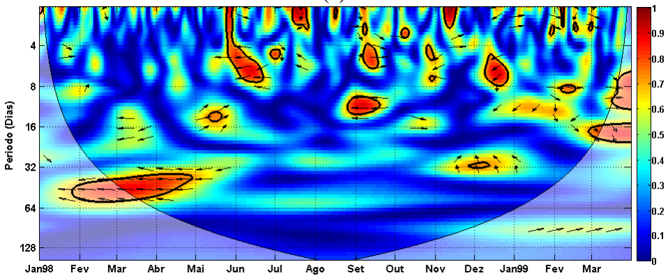
Figura 4.10 - Como na Fig. 4.7, mas para ondeleta cruzada entre a AROLE não-filtrada em um ponto no centro-oeste do Pacífico sul tropical e a AROLE não-filtrada em um ponto na área sul da ZCAS.
