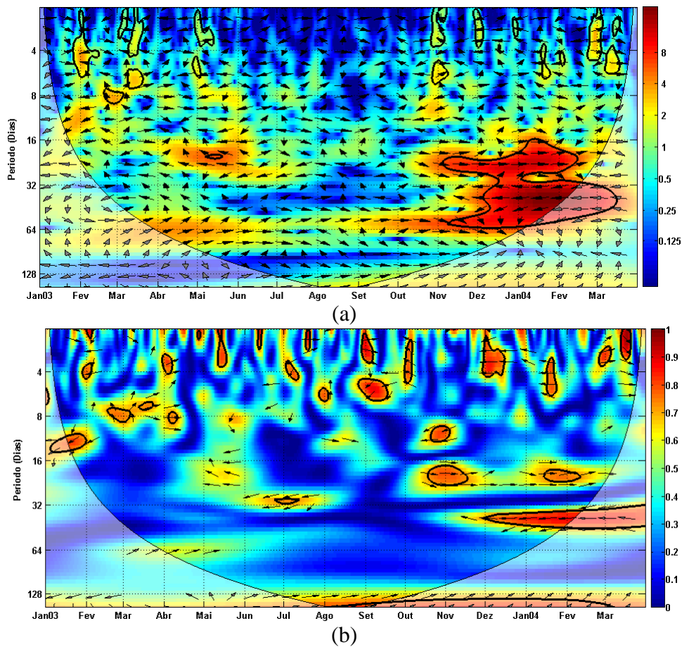
Figura 4.45 - Como na Fig. 4.7, mas para ondebata cruzada entre a AROLE não-filtrada em um ponto no oeste do Pacífico equatorial e a AROLE não-filtrada em um ponto na área norte da ZCAS.
