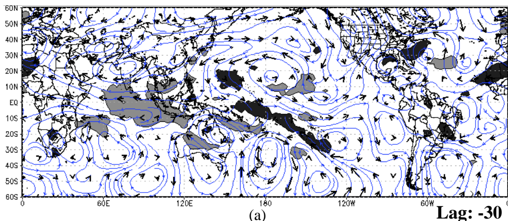
Figura 4.3 - Composições dos 28 eventos para as anomalias de ROLE (sombreado), linha de corrente e vetor vento em 200 hPa filtradas em 30-60 dias em defasagens de (a) -30 dias; (b) -25 dias; (c) -20 dias; (d) -15 dias; (e) -10 dias; (f) -5 dias; e (g) 0 dia antes do início de cada evento. Apenas AROLE mais positivas (negativas) do que 2 (-2) W/m^2 são mostradas em sombreado escuro (claro). (Continua).
