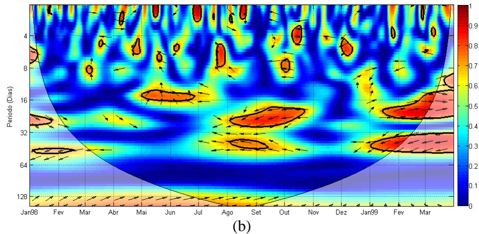
Figura 4.12 - Como na Fig. 4.7, mas para ondeleta cruzada entre a AROLE não-filtrada em um ponto no centro-oeste do Pacífico sul subtropical e a AROLE não-filtrada em um ponto na área sul da ZCAS.
