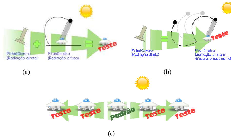
Figura 2 - (a) Calibração por comparação utilizando um pirheliômetro de referência para irradiância solar direta e um piranômetro de referência para irradiância difusa; (b) Por comparação utilizando um pirheliômetro de referência, o Sol como fonte de radiação e um disco sombreador removível para o piranômetro; e (c) Por comparação com um piranômetro de referência, utilizando o Sol como fonte, sob condições naturais de exposição.
