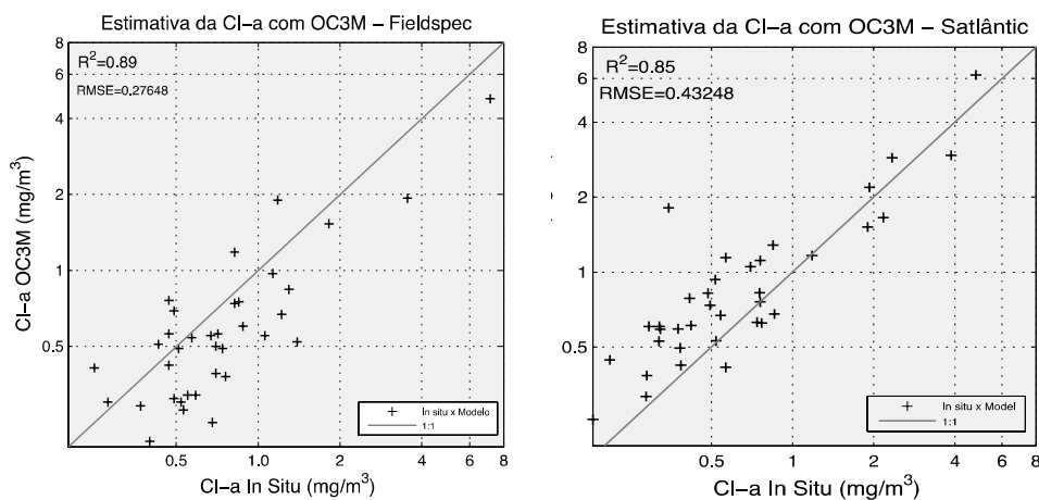
Figura 4.26: Resultados dos testes do modelo OC3M com os dados do Fieldspec (esquerda) e Satlântic (direita), com a Cl a in situ no eixo horizontal e a Cl a ( \text{mg}/\text{m}^3 ) modelada no eixo vertical.
