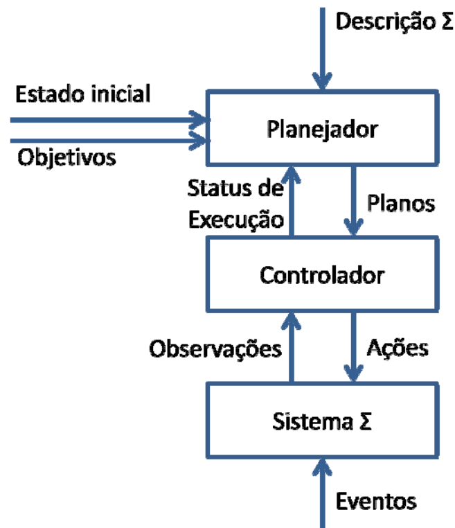
Figura 2.5 - Modelo conceitual de planejamento Fonte: Ghallab, Nau e Traverso (2004)
